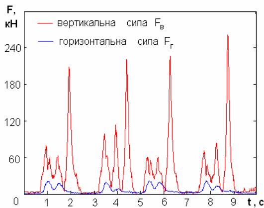
Рис. 3. Дія коліс тепловоза на рейку при русі в кривій радіусом 300 м
