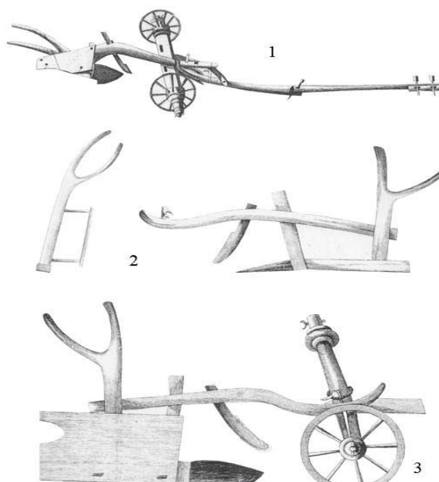
Рис. 3. Из описаний плугов И.А. Гюльдешедта: 1 – плуг из Черниговской губернии; 2, 3 – грузинские плуги
