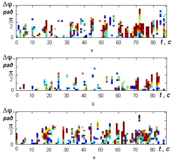
Рис. 4. Зміна зсуву фаз реєстрованої акустичної емісії першим радіочастотним акустичним датчиком відносно акустичної емісії, реєстрованої трьома іншими датчиками
