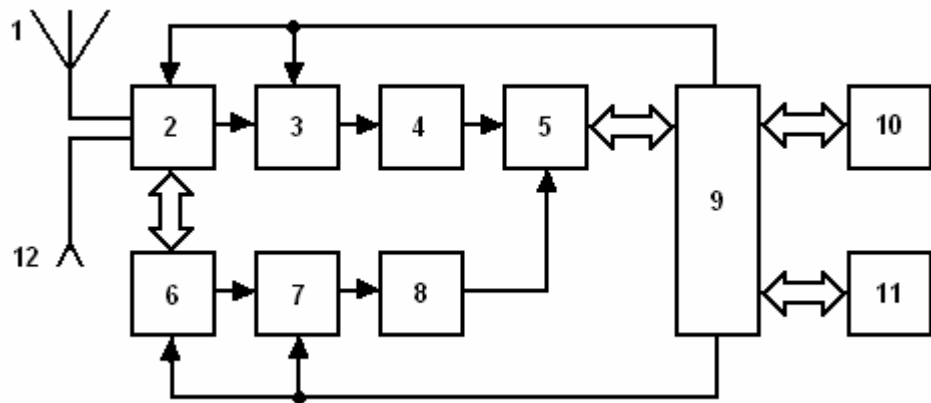
Рис. 2. Блок-схема системи збору даних радіочастотних датчиків: 1 – широкопasmова антена; 2 – скануючий приймач; 3 – частотний детектор; 4 – підсилювач низької частоти; 5 – багатоканальний АЦП; 6 – частотний аналізатор спектра, що містить синхрогенератор; 7 – фазовий аналізатор; 8 – нормуючий перетворювач; 9 – мікроконтролер; 10 – пристрої керування процесами й автоматики; 11 – сигналізуючий пристрій; 12 – вхід коаксіальної мережі системи збору даних
