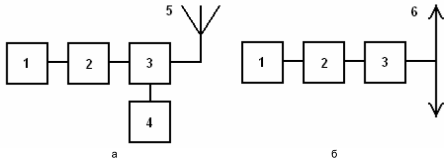
Рис. 1. Блок-схема радіочастотного акустичного датчика: а – незалежне електроживлення і передача даних по радіоканалу; б – електроживлення і передача даних по коаксіальному кабелю: 1 – протектор, що погоджує акустичні середовища об'єкт контролю – коливальний контур; 2 – реактивна ємність котушки індуктивності нелінійного коливального контуру; 3 – автогенератор з ємнісним або індуктивним зворотним зв'язком; 4 – автономне джерело електроживлення; 5 – укорочена резонансна антена; 6 – коаксіальний кабель системи збору інформації і електроживлення радіочастотних датчиків
