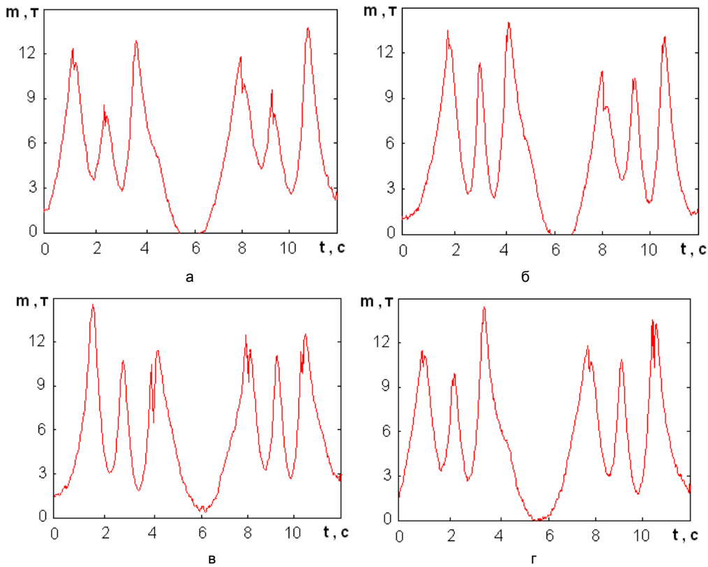
Рис. 2. Графіки вертикальної сили, що діє на рейку з боку коліс тепловозних секцій, наведені в одиницях маси: а – тепловоз 2ТЕ116 №644 секція А; б – тепловоз 2ТЕ116 №895 секція А; в – тепловоз 2ТЕ116 №947 секція Б; г – тепловоз 2ТЕ116 №1077 секція А
