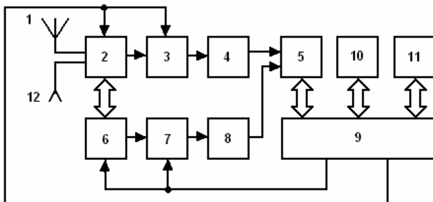
Рис. 1. Блок-схема системи контролю і керування протяжним об'єктом на основі радіочастотних датчиків: 1 – широкопasmова антена; 2 – скануючий приймач; 3 – частотний детектор; 4 – підсилювач низької частоти; 5 – багатоканальний АЦП; 6 – частотний аналізатор спектра, що містить синхрогенератор; 7 – фазовий аналізатор; 8 – нормуючий перетворювач; 9 – мікроконтролер; 10 – пристрої керування процесами й автоматики; 11 – сигналізуючий пристрій; 12 – вхід коаксіальної мережі системи збору даних
