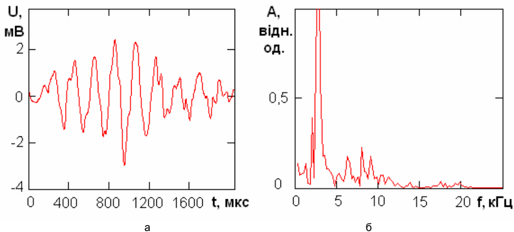
Рис. 1. Параметри електромагнітної емісії: а – електричний сигнал; б – спектр сигналу
