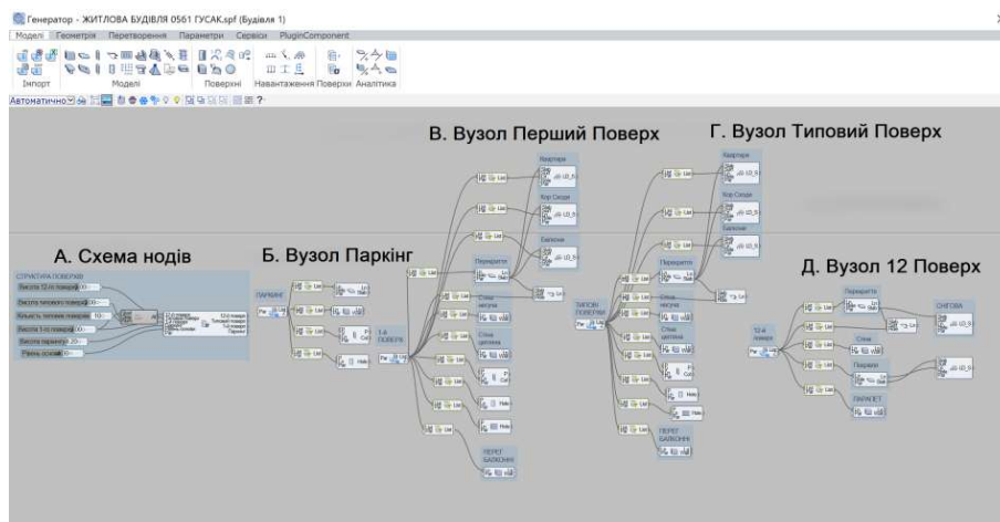
Рис. 4. Блок-схема будівлі у генераторі вузлів
