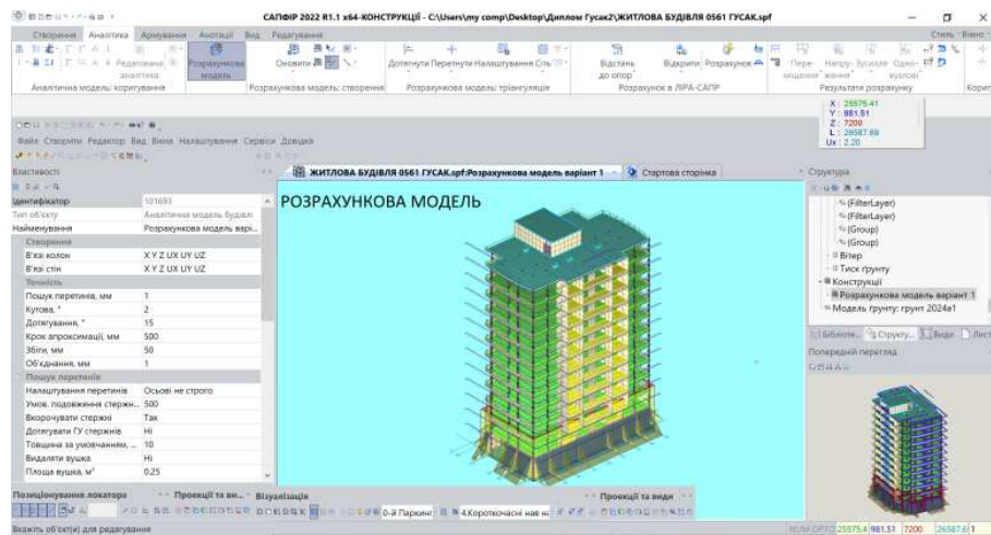
Рис. 3. Розрахункова модель будівлі
