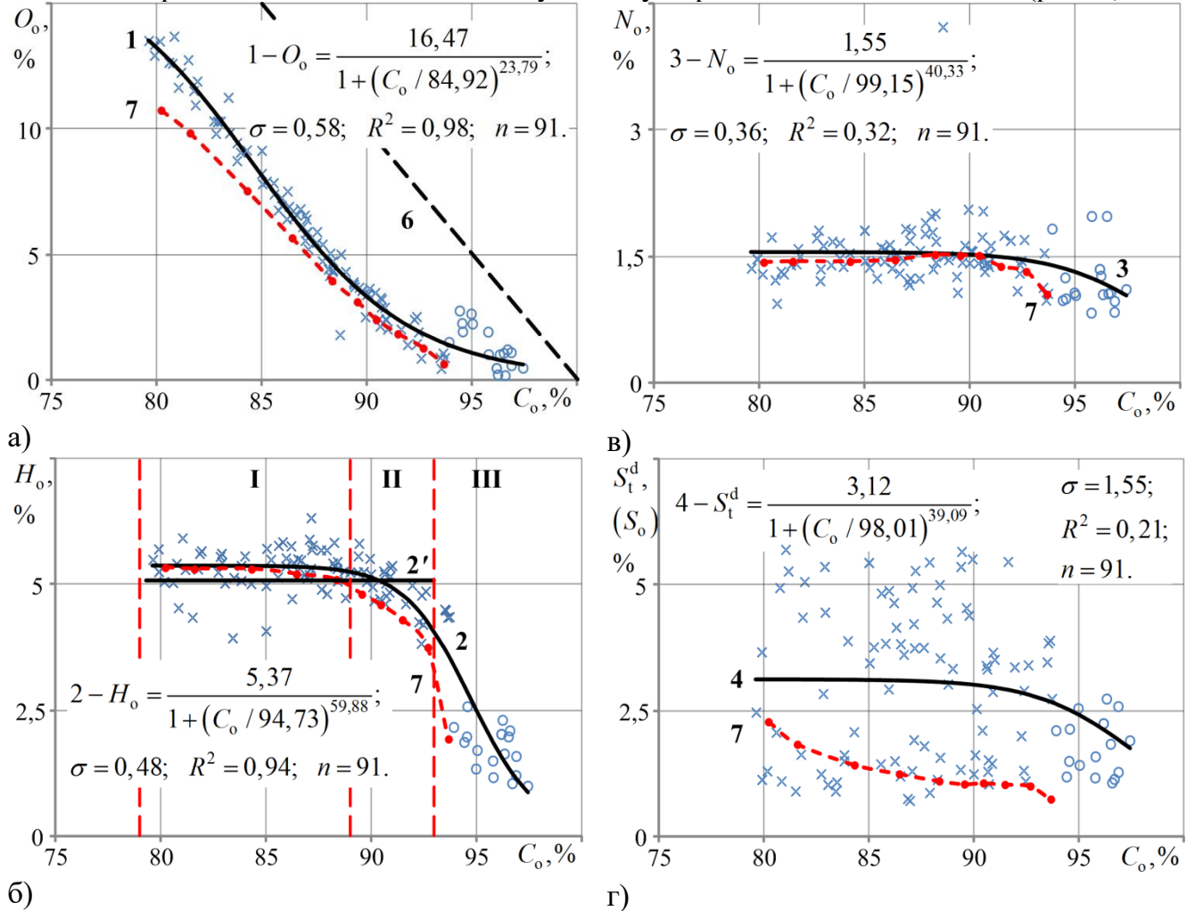
Рисунок 1. Якісні показники споживчих властивостей вугілля за результатами обробки лабораторних та аналітичних проб згідно [1] для шахтопластів Донбасу та їх залежності на умовну органічну масу від вмісту вуглецю ( C_o ): а) кисню ( O_o ); б) водню ( H_o ); в) азоту ( N_o ); г) загальної сірки ( S_t^d ): 1, 2, 3, 4, 5 - усереднені криві залежностей відповідно кисню (1), водню (2), азоту (3), загальної сірки (4); 2' - середній вміст водню ( \bar{H}_o = 5,09\% ) для кам'яновугільних шахтопластів при C_o < 93\% ; 6 - залежність \Sigma O_o, H_o, N_o від C_o , прийнята за розрахункового визначення O_o [1]; 7 - усереднені залежності середнього складу вугілля, у тому числі вмісту сірки органічної маси S_o (г), для шахтопластів Донецького басейну [2];
