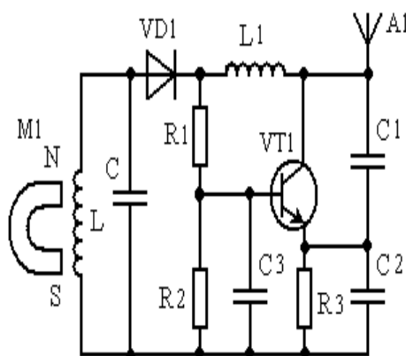
Рис. 2. Принципиальная схема устройства контроля колеса
