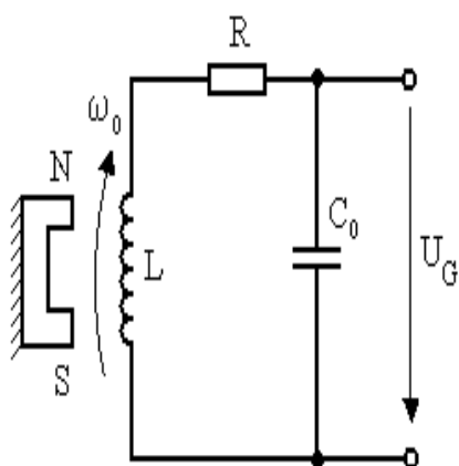
Рис. 2. Эквивалентная схема магнитоэлектрического генератора с емкостной нагрузкой
