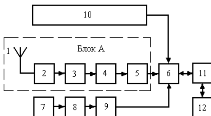
Рис. 3. Блок-схема напольного устройства мониторинга технического состояния колес электропоезда: 1 – приемная рупорная СВЧ антенна; 2 – малозумящий полосовой усилитель; 3 – усилитель-ограничитель; 4 – амплитудный детектор; 5 – формирователь импульсов; 6 – микроконтроллер; 7 – шлейфовый датчик счета осей колесных пар; 8 – усилитель; 9 – формирователь импульсов; 10 – блок регистрации СВЧ сигнала с поверхности колеса (аналогичный блоку А); 11 – радиомодем; 12 – информационная сеть
