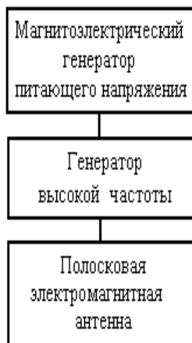
Рис. 3. Блок-схема устройства контроля бандажа и колесного центра
