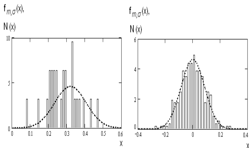
Рис. 1. Щільність імовірності і гістограма частоти
