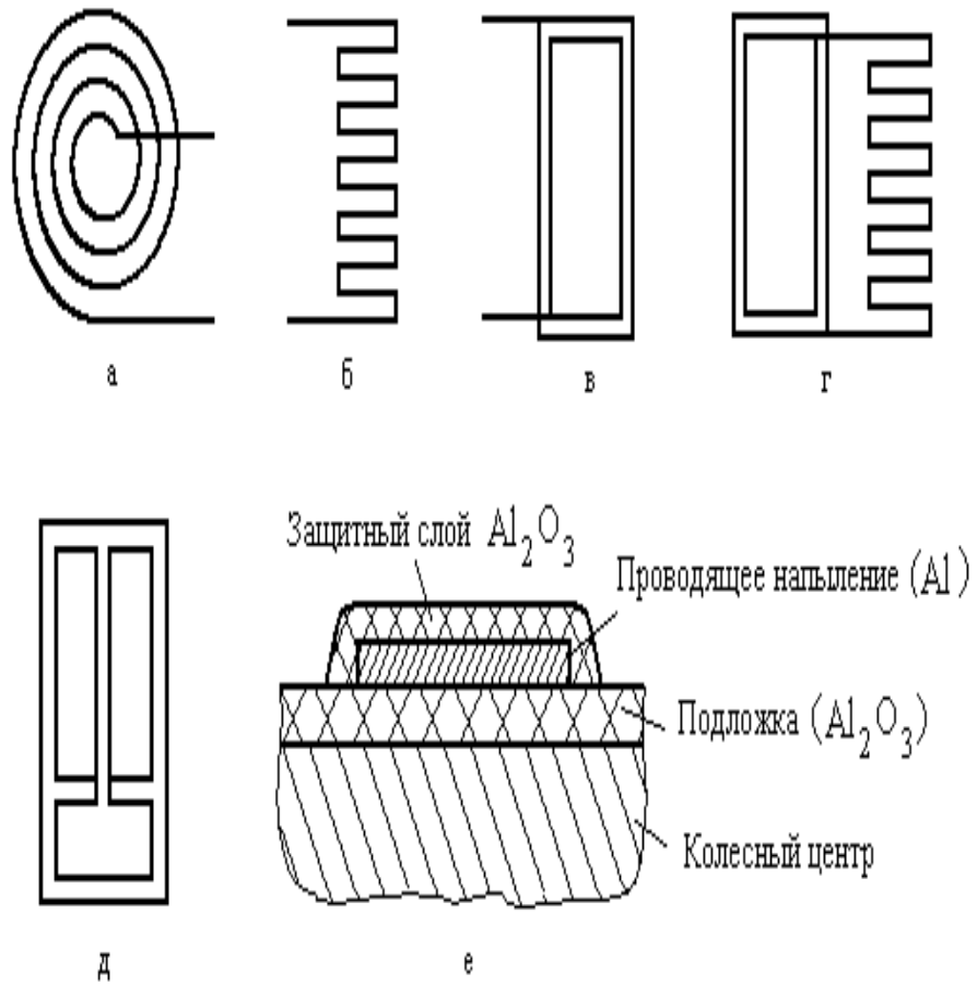
Рис. 1. Схемы исполнения элементов датчиков устройства контроля напылением: а – электромагнит; б – индуктивность; в – емкость; г – колебательный контур; д – полосковый LC-контур; е – технология нанесения слоев
