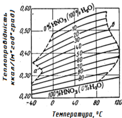
Рис. 1.13. Залежність теплопровідності водних розчинів нітратної кислоти від температури при різних масових концентраціях \text{HNO}_3
