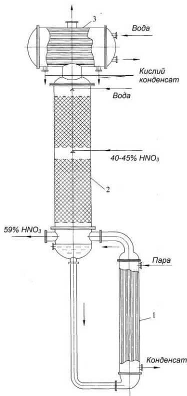
Рис. 5.13. Схема установки попереднього концентрування ННК: 1 – кип'ятильник; 2 – ректифікаційна колона; 3 – конденсатор
