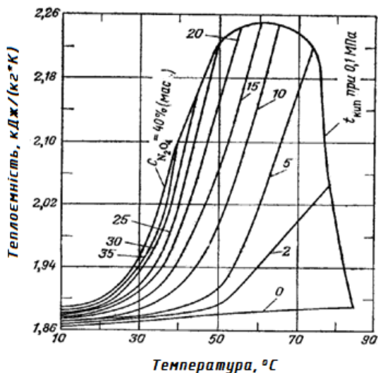
Рис. 1.25. Залежність ізобарної теплоємності розчинів \text{HNO}_3\text{--N}_2\text{O}_4 від температури при різних масових вмістах оксиду нітрогену (IV)
