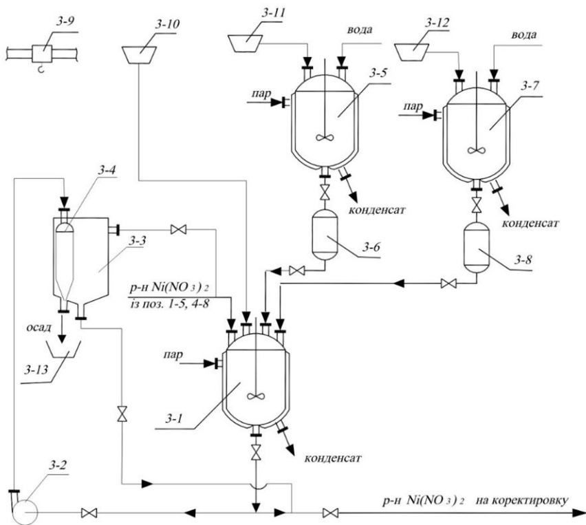
Рис. 6.12. Технологічна схема очищення розчину нітратів металів від домішок \text{Fe}^{3+} і \text{SO}_4^{2-} :
