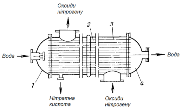
Рис. 5.35. Головний холодильник: 1, 4 — кришки; 2 — корпус; 3 — труби
