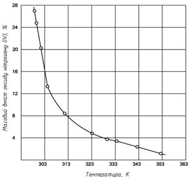
Рис. 3.22. Залежність масового вмісту оксиду нітрогену (IV) в кубовому розчині від температури
