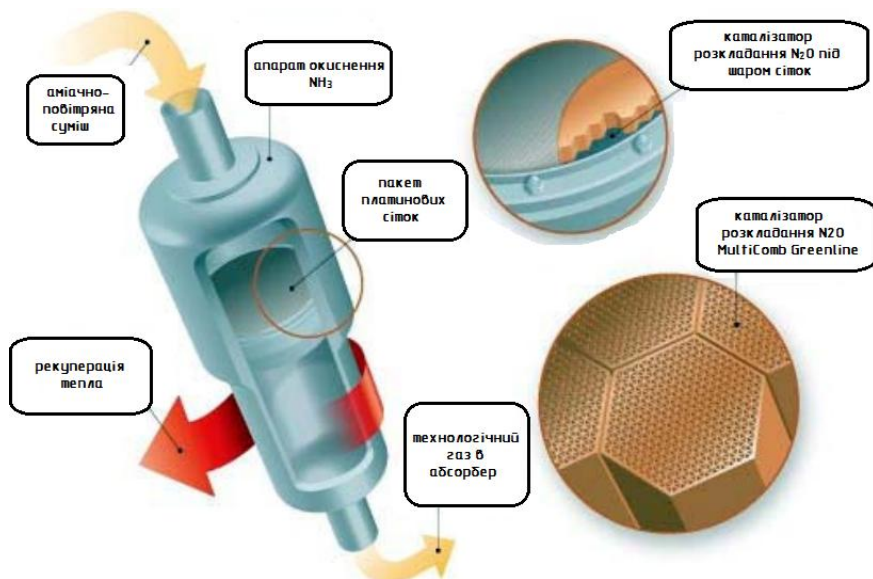
Рис. 5.5. Принципова схема контактного апарату окиснення аміаку з вторинним блоковим катализатором розкладання оксиду динітрогену
