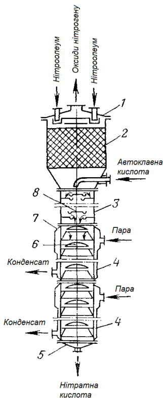
Рис. 5.32. Відбілювальна колона:
