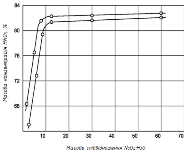
Рис. 3.20. Залежність масової концентрації HNO_3 у кубовому розчині ректифікаційної колони від вихідного масового співвідношення N_2O_4:H_2O при різних початкових концентраціях HNO_3 , % мас: 1 – 40; 2 – 50
