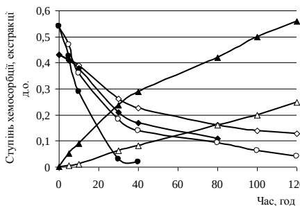
Рис. 6.2. Динаміка зміни ступеня екстракції Ni^{2+} і хемосорбції NO_x в системі з каталізатором НКМ-1
