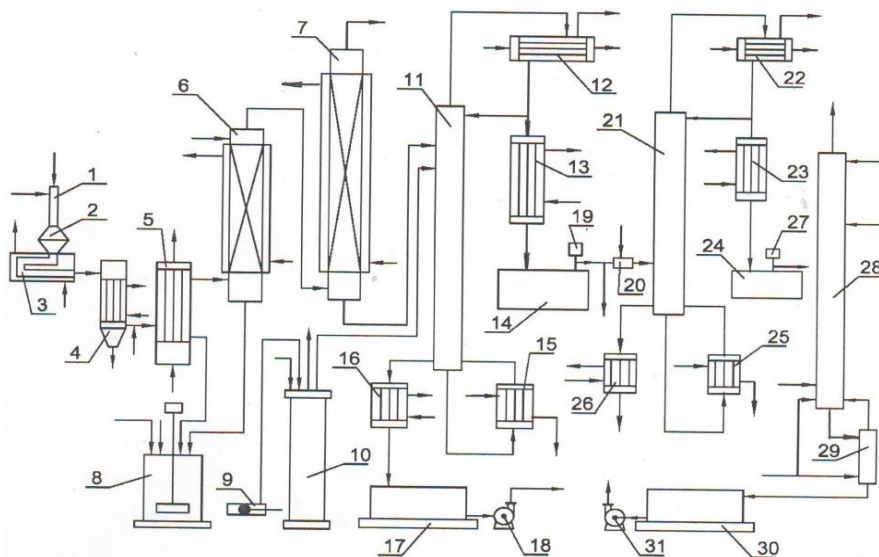
Рис. 5.7. Принципова технологічна схема отримання рідких сумішей N_2O_3-N_2O_4 з водних розчинів нітратної кислоти та оксидів нітрогену
