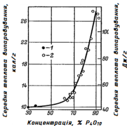
Рис. 1.40. Залежність теплоти випаровування від концентрації P_4O_{10} в системі P_2O_5-H_2O : 1 – за даними (Hartley, Holmes, Jacques, Mole & McCoubrey, 1963); 2 – за даними (Broun & Whitt, 1952)
