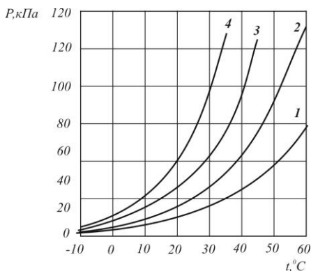
Рис. 3.53. Залежність тиску насиченої пари в системі \text{HNO}_3\text{--N}_2\text{O}_5\text{--N}_2\text{O}_4 від температури при вмісті \text{N}_2\text{O}_4 5% і концентраціях \text{N}_2\text{O}_5 , %: 1 – 0; 2 – 10; 3 – 20; 4 – 30
