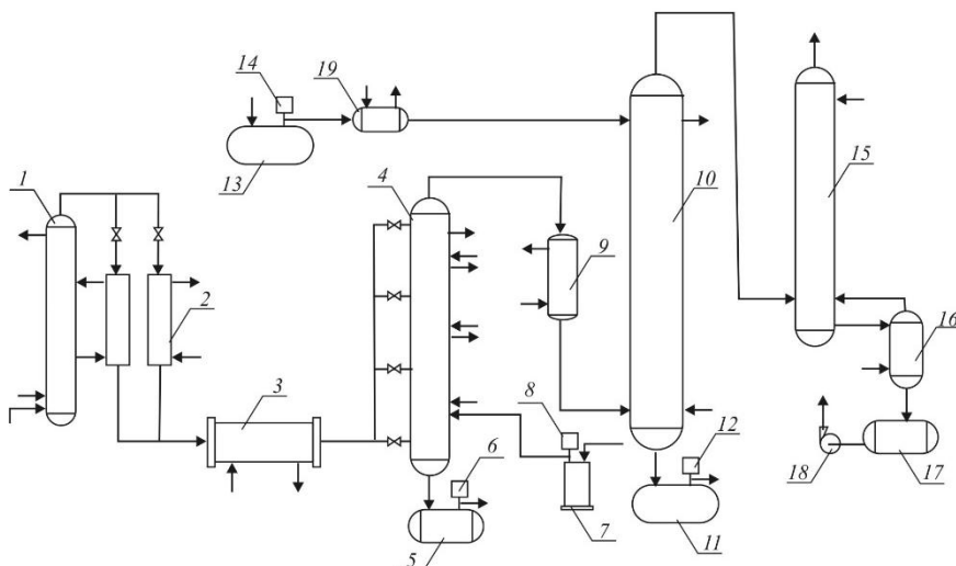
Рис. 5.10. Принципова технологічна схема газорідинного окиснення оксиду нітрогену (IV) озono-кисневою сумішшю і поглинання \text{N}_2\text{O}_5 концентрованою нітратною кислотою:
