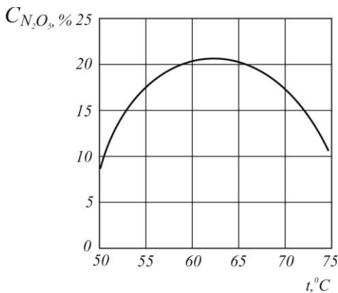
Рис. 3.61. Залежність вмісту N 2 O 5 в дистиляті від температури флегми
