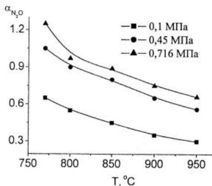
Рис. 4.8. Залежність ступеня окиснення \text{NH}_3 в \text{N}_2\text{O} від температури
