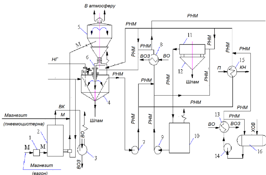
Рис. 5.23. Установка приготування розчинів нітрату магнію:
