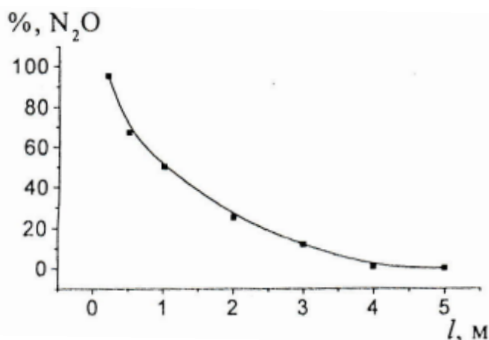
Рис. 4.3. Залежність відносного вмісту \text{N}_2\text{O} в нітрозному газі від відстані від каталізаторних сіток (лінійна швидкість – 2,2 м/с; T = 890^\circ\text{C} )
