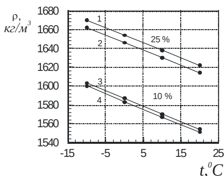
Рис. 3.30. Залежність густини розчинів HNO_3-N_2O_5-N_2O_4 від температури при сумарному масовому вмісті оксидів нітрогену, рівних 10 і 25%, і масових співвідношеннях N_2O_5:N_2O_4 : 1 – 30:1; 2 – 1:1; 3 – 1:1; 4 – 30:1
