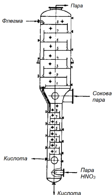
Рис. 5.26. Колона ректифікації сокової пари
