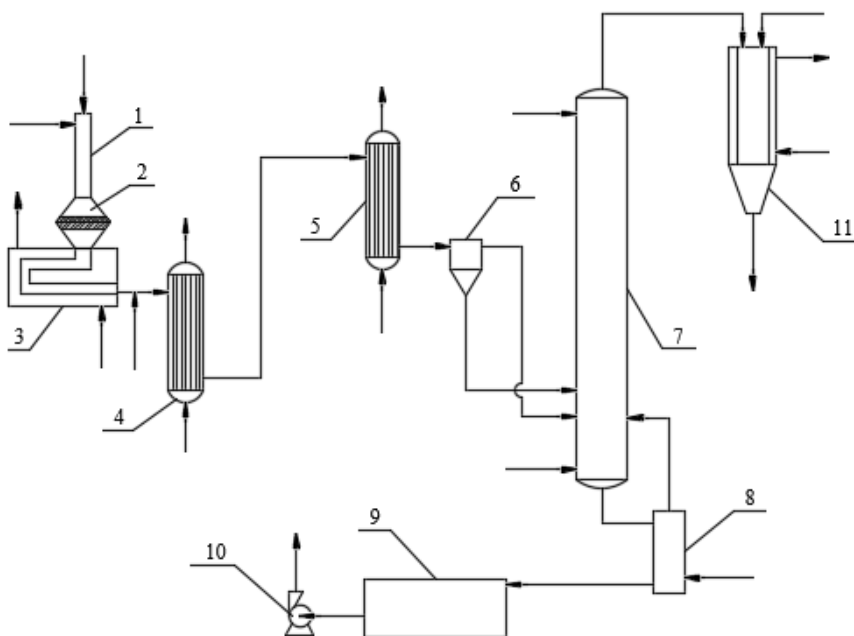
Рис. 5.6. Принципова технологічна схема виробництва неконцентрованої нітратної кислоти з відновленням оксиду динітрогену: 1 – змішувач; 2 – контактний апарат; 3 – котел-утилізатор; 4 – холодильник-окиснювач; 5 – конденсатор; 6 – сепаратор; 7 – абсорбційна колона; 8 – продувна колона; 9 – збірник продукційної нітратної кислоти; 10 – насос; 11 – реактор відновлення оксидів нітрогену
