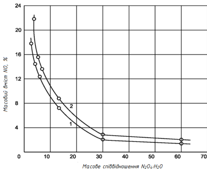
Рис. 3.19. Залежність масового вмісту NO в дистилаті від вихідного масового співвідношення N_2O_4:H_2O при різних початкових масових концентраціях HNO_3 : 1 – 50; 2 – 40
