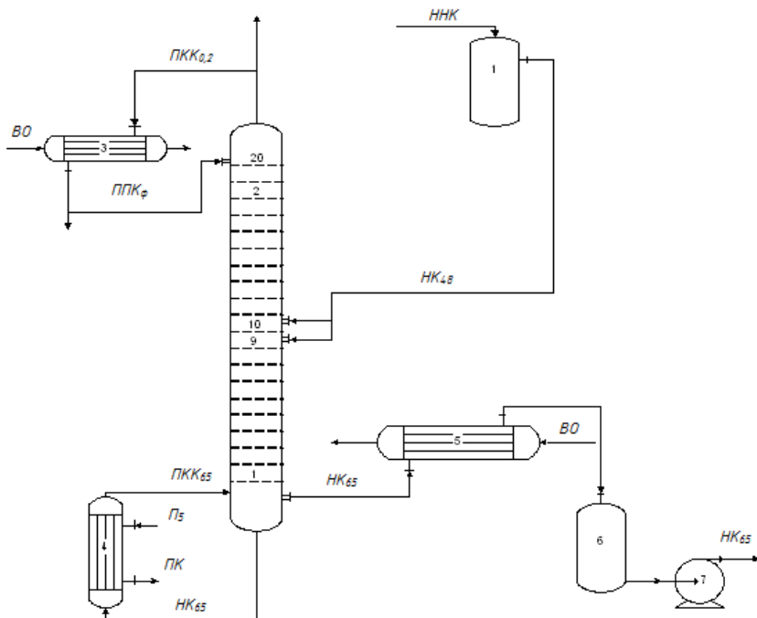
Рис. 5.14. Схема установки попереднього концентрування доазеотропної нітратної кислоти:
