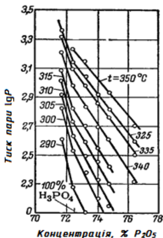
Рис. 1.39. Залежність логарифму тиску пари в системі P_2O_5-H_2O від концентрації P_2O_5 при різних температурах
