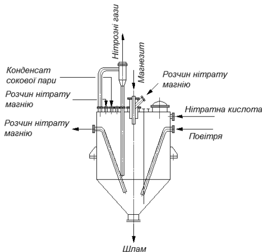
Рис. 5.28. Ємність для розчинення магнезиту
