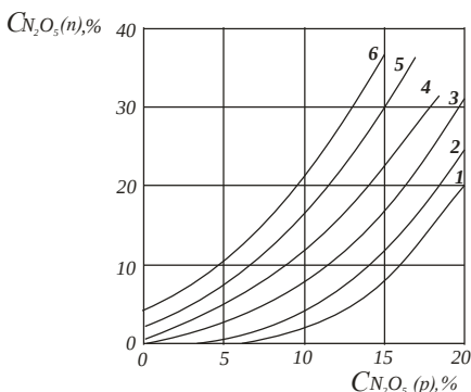
Рис. 3.55. Діаграма фазової рівноваги рідина – пара бінарної системи \text{HNO}_3\text{--N}_2\text{O}_5 при температурах, ^{\circ}\text{C} : 1 – (-20); 2 – 0; 3 – 20; 4 – 40; 5 – 60; 6 – 80
