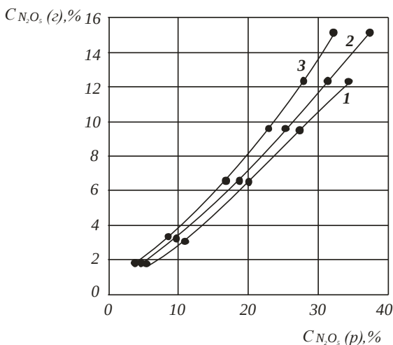
Рис. 3.35. Залежність концентрації \text{N}_2\text{O}_5 в газовій фазі від його вмісту в рідкій фазі при температурах, °C: 1 – (-10); 2 – 0; 3 – 10
