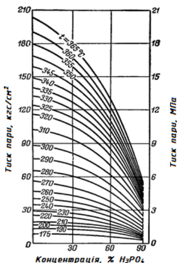
Рис. 1.37. Залежність тиску насиченої пари над розчинами P_2O_5-H_2O від концентрації фосфатної кислоти при різних температурах
