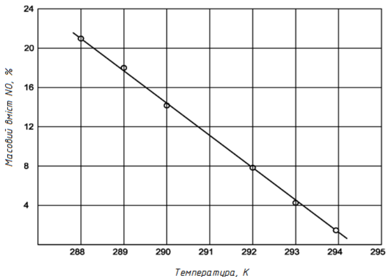
Рис. 3.21. Залежність масового вмісту NO в дистилаті від температури флегми
