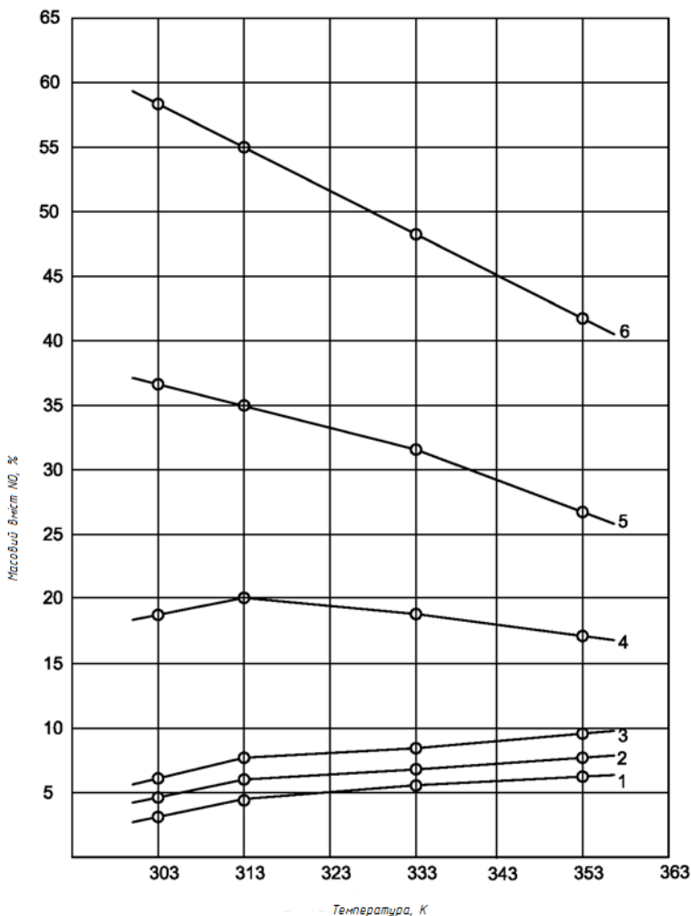
Рис. 3.14. Залежність масового вмісту NO в паровій фазі від температури при початковій концентрації HNO_3 40% мас. та різних масових співвідношеннях N_2O_4:H_2O : 1 – 12:1; 2 – 6:1; 3 – 4:1; 4 – 2:1; 5 – 1:1; 6 – 1:2
