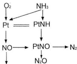
Рис. 4.12. Схема реакції окиснення аміаку на платиноїдному каталізаторі
