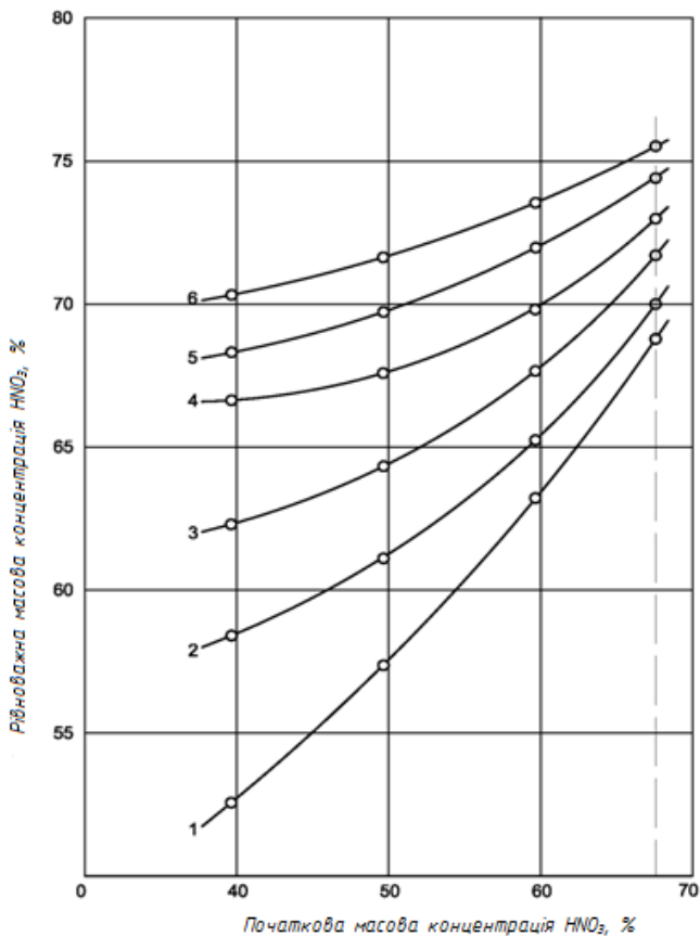
Рис. 3.10. Залежність рівноважної масової концентрації HNO_3 від початкової масової концентрації HNO_3 при різних масових співвідношеннях N_2O_4:H_2O : 1 – 1:2; 2 – 1:1; 3 – 2:1; 4 – 4:1; 5 – 6:1; 6 – 12:1
