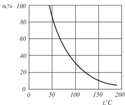
Рис. 3.38. Залежність ступеня використання озону ( \alpha ) від температури процесу в реакторі
