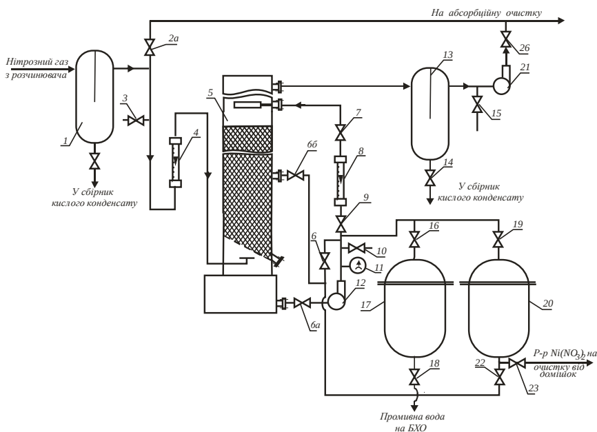
Рис. 6.7. Схема дослідно-промислової установки хемосорбції оксидів нітрогену й екстракції металів з відпрацьованих механічно міцних каталізаторів:
