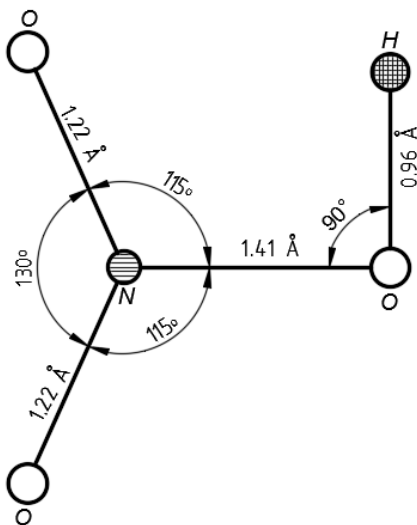
Рис. 1.1. Будова молекули \text{HNO}_3
