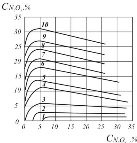
Рис. 3.28. Лінії постійного значення окиснювально-відновного потенціалу розчинів \text{HNO}_3\text{--N}_2\text{O}_5\text{--N}_2\text{O}_4 при 20^\circ\text{C} , мВ:
