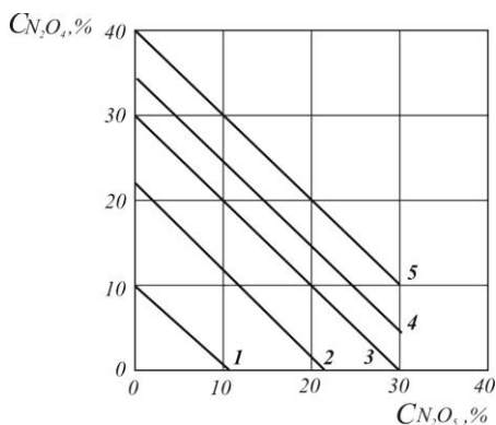
Рис. 3.52. Лінії постійного значення тиску насиченої пари (ізобари) розчинів \text{HNO}_3\text{--N}_2\text{O}_5\text{--N}_2\text{O}_4 при 30^\circ\text{C} , кПа: 1 – 20; 2 – 40; 3 – 60; 4 – 80; 5 – 100
