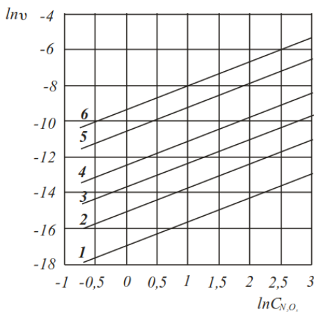
Рис. 3.45. Залежність швидкості розпаду розчинів \text{HNO}_3\text{--N}_2\text{O}_5 від концентрації \text{N}_2\text{O}_5 при температурах, ^{\circ}\text{C} : 1 – 20; 2 – 30; 3 – 40; 4 – 50; 5 – 60; 6 – 70
