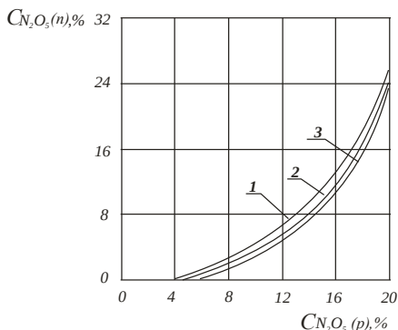
Рис. 3.56. Залежність вмісту \text{N}_2\text{O}_5 в паровій фазі від його концентрації в рідині при 0^{\circ}\text{C} і вмісту \text{N}_2\text{O}_4 , %: 1 – 0; 2 – 2; 3 – 5
