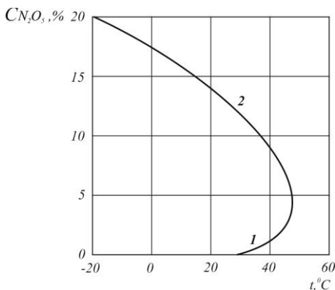
Рис. 3.54. Залежність складу азеотропів від температури: 1 — з максимумом тиску; 2 — з мінімумом тиску
