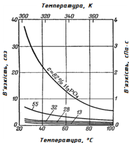
Рис. 1.34. Залежність динамічної в'язкості розчинів \text{H}_3\text{PO}_4\text{--H}_2\text{O} від температури при різних концентраціях \text{H}_3\text{PO}_4
