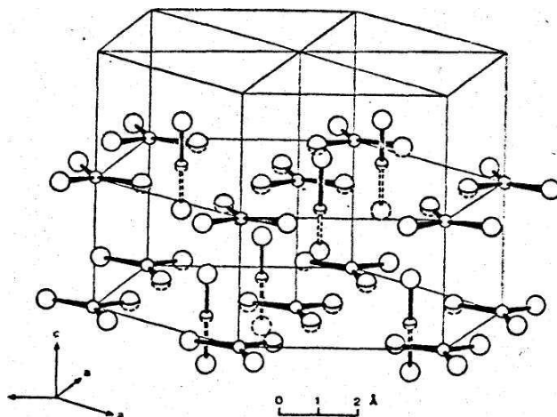
Рис. 1.30. Будова кристалічного пентаоксиду динітрогену ( 1 \text{ \AA} = 0,1 \text{ нм} )
