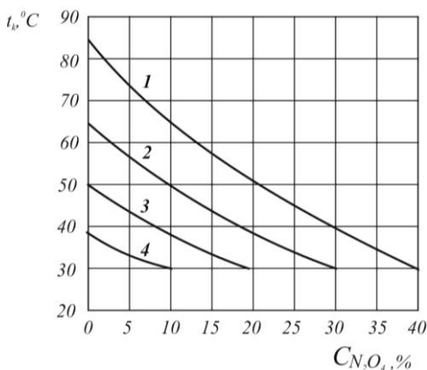
Рис. 3.47. Залежність температури кипіння розчинів \text{HNO}_3\text{--N}_2\text{O}_5\text{--N}_2\text{O}_4 від концентрації \text{N}_2\text{O}_4 при вмісті \text{N}_2\text{O}_5 , %: 1 – 0; 2 – 10; 3 – 20; 4 – 30
