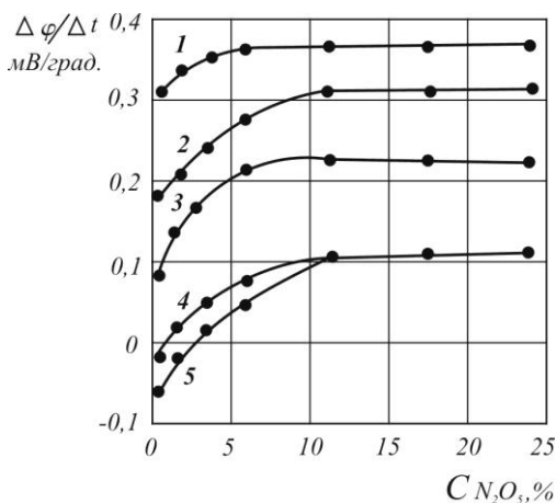
Рис. 3.27. Залежність температурного коефіцієнта ( \Delta\phi/\Delta t ) окиснювально-відновного потенціалу розчинів HNO_3-N_2O_5-N_2O_4 від масової концентрації N_2O_5 при масовому вмісті N_2O_4 , %: 1 – 0,01; 2 – 1; 3 – 2; 4 – 5; 5 – 10
