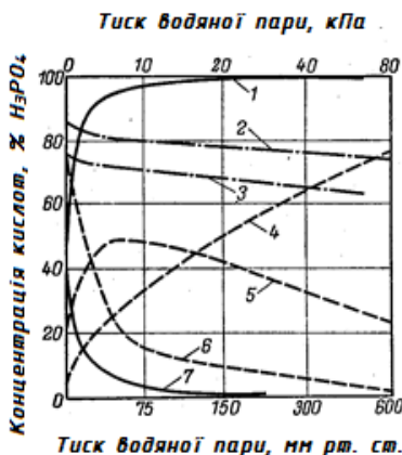
Рис. 1.41. Залежність складу фосфатних кислот від тиску водяної пари при 423 та 523 К: 1 – \text{H}_3\text{PO}_4 (423 К); 2 – \text{P}_2\text{O}_5 (523 К); 3 – \text{P}_2\text{O}_5 (423 К); 4 – \text{H}_3\text{PO}_4 (523 К); 5 – \text{H}_4\text{P}_2\text{O}_7 (523 К); 6 – \text{HPO}_3 (523 К); 7 – \text{H}_4\text{P}_2\text{O}_7 (423 К)
