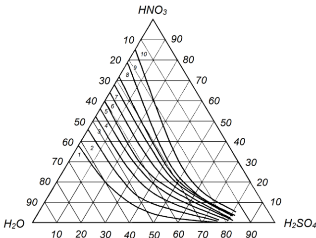
Рис. 5.15. Рівноважні концентрації нітратної кислоти у парі над сумішшю \text{HNO}_3\text{--H}_2\text{O--H}_2\text{SO}_4 , % мас:
