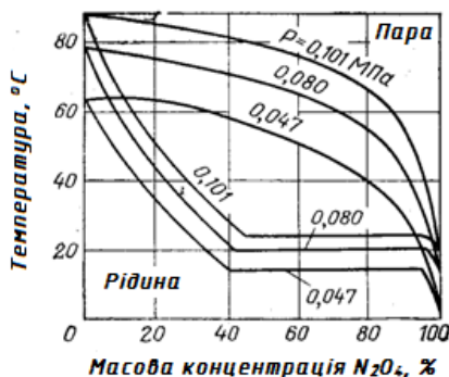
Рис. 1.21. Діаграма кипіння розчинів \text{HNO}_3\text{--N}_2\text{O}_4 при різних тисках
