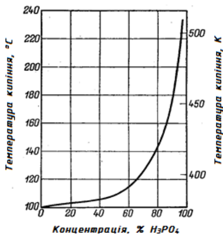
Рис. 1.35. Залежність температури кипіння розчинів \text{H}_3\text{PO}_4\text{--H}_2\text{O} від концентрації фосфатної кислоти
