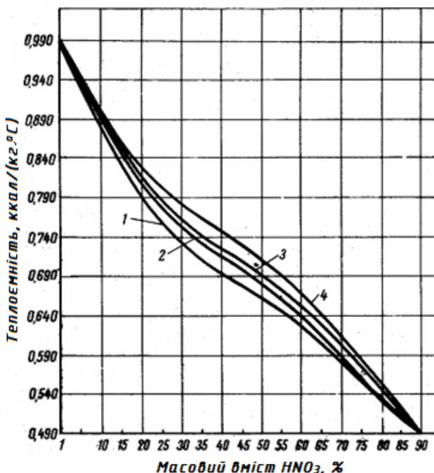
Рис. 1.10. Залежність теплоємності від масового вмісту нітратної кислоти в системі \text{HNO}_3\text{--H}_2\text{O} при різних температурах ( ^{\circ}\text{C} ): 1 – 2,53; 2 – 21,07; 3 – 39,49; 4 – 61,11
