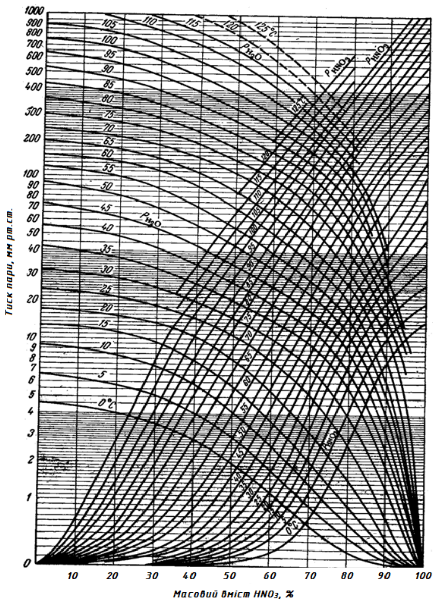
Рис. 1.6. Залежність парціальних тисків \text{HNO}_3 і \text{H}_2\text{O} над водними розчинами нітратної кислоти при різних температурах
