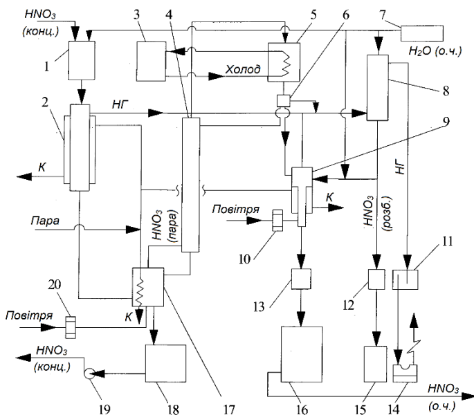
1 – напірний бак; 2 – дегазатор; 3 – холодильна установка; 4 – колона псевдоректифікації; 5 – конденсатор; 6 – розподільник; 7 – ємність (напірний бак); 8 – колона абсорбції; 9 – апарат для розведення; 10, 20 – фільтри; 11 – нейтралізатор; 12, 13 – збірники; 14 – вакуум-насос; 15 – відділення хімічної обробки бутлів; 16 – відділення розливу товарної кислоти; 17 – випарник; 18 – бак дренажний; 19 – насос; НГ – нітрозний газ; К – конденсат; о.ч. – особливої чистоти; конц. – концентрована; розб. – розбавлена
