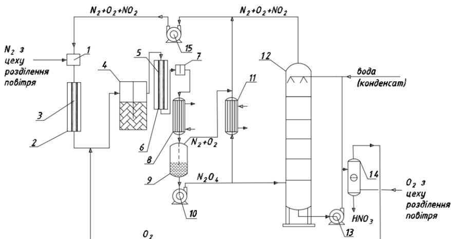
Рис. 5.42. Технологічну схему фотохімічного виробництва неконцентрованої нітратної кислоти окисненням N_2 :
