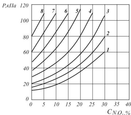
Рис. 3.51. Залежність тиску насиченої пари системи \text{HNO}_3\text{--N}_2\text{O}_5\text{--N}_2\text{O}_4 від концентрації \text{N}_2\text{O}_5 при 30 °С і вмісті \text{N}_2\text{O}_4 , %: 1 – 0; 2 – 5; 3 – 10; 4 – 15; 5 – 20; 6 – 25; 7 – 30; 8 – 35
