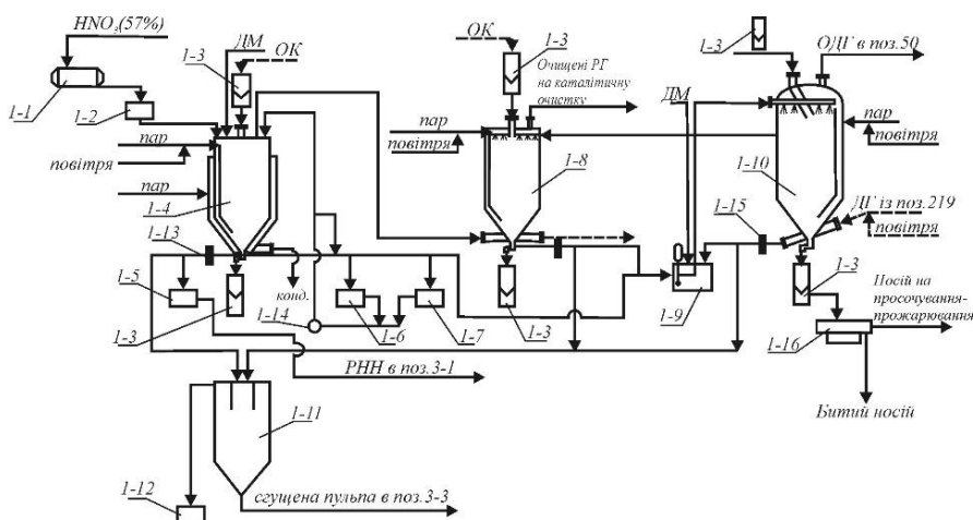
Рис. 6.10. Технологічна схема сумішеного процесу хемосорбції оксидів нітрогену та екстракції металів з механічно міцних каталізаторів:
