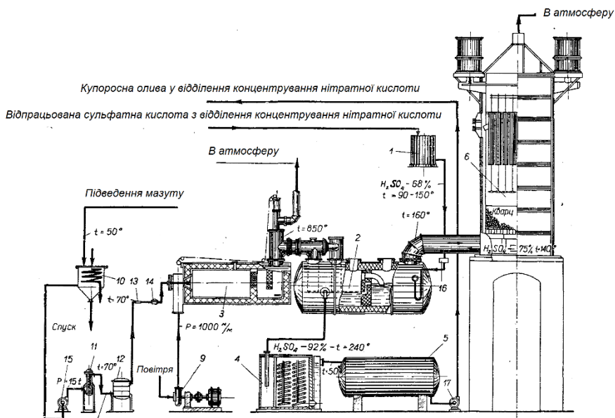
Рис. 5.19. Принципова схема концентрування сульфатної кислоти:
