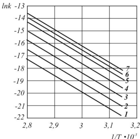
Рис. 3.44. Залежність константи швидкості розпаду від температури при масових концентраціях нітратної кислоти, %: 1 – 95; 2 – 96; 3 – 97; 4 – 98; 5 – 99; 6 – 99,5; 7 – 100
