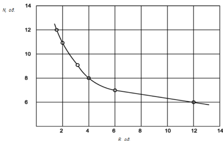
Рис. 3.15. Залежність числа теоретичних тарілок ( N ) від флегмового числа ( R )
