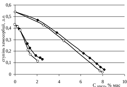
Рис. 6.3. Залежність \alpha_{NO_x} від концентрації HNO_3 при різних C_{NO_x}^{noch} в системі з каталізатором НКМ-1 і на інертній насадці
