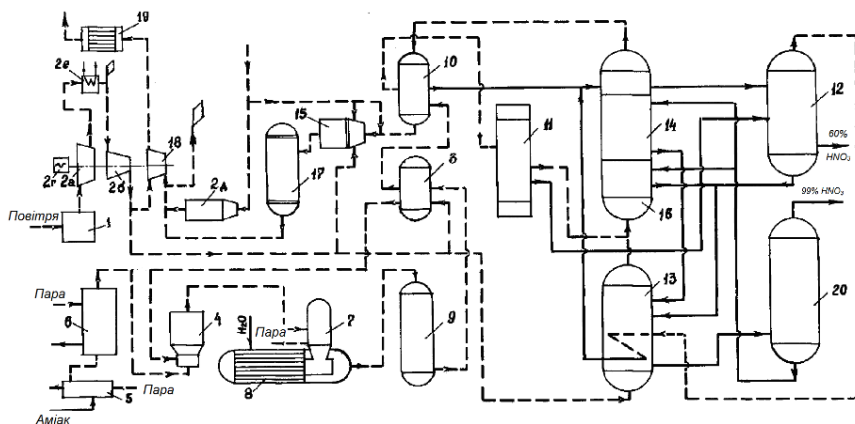
Рис. 5.29. Принципова технологічна схема виробництва концентрованої нітратної кислоти через кислоту проміжної концентрації:
