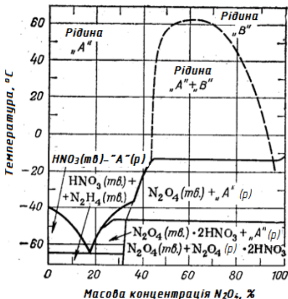
Рис. 1.24. Діаграма стану системи \text{HNO}_3\text{--N}_2\text{O}_4 при тиску 0,1013 МПа
