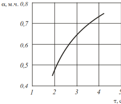
Рис. 3.39. Залежність ступеня поглинання ( \alpha ) N_2O_5 нітратною кислотою від часу контакту газової і рідкої фаз при 0^\circ\text{C} і лінійній швидкості газу 0,2 м/с
