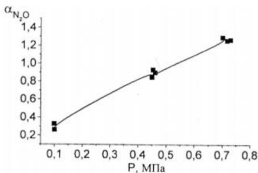
Рис. 4.9. Залежність ступеня окиснення \text{NH}_3 в \text{N}_2\text{O} від тиску
