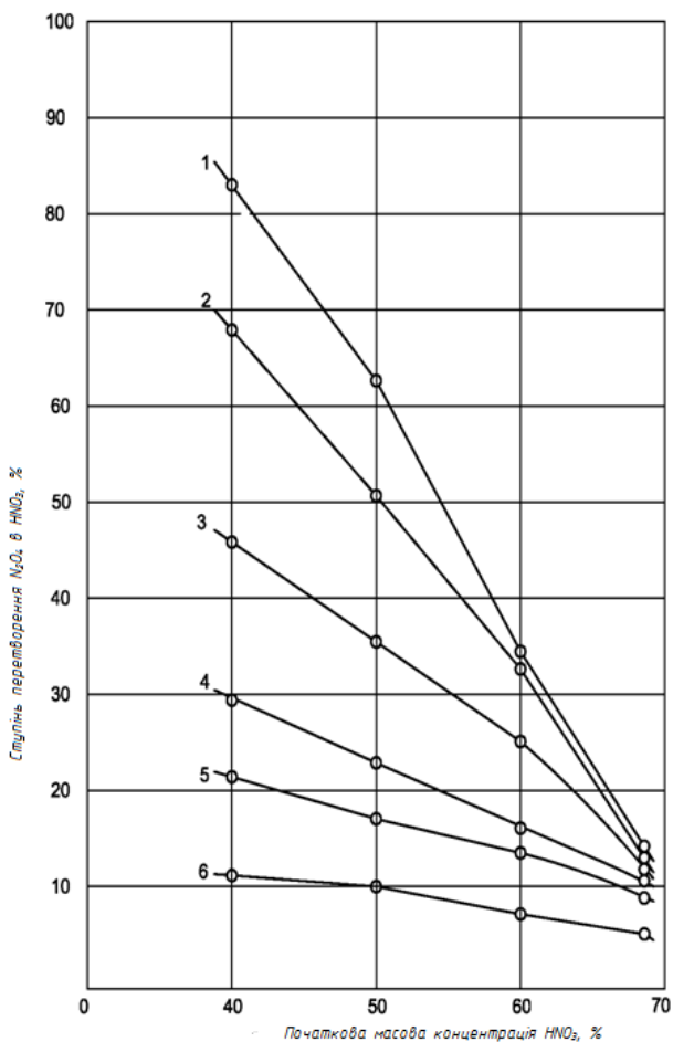
Рис. 3.11. Залежність ступені перетворення \text{N}_2\text{O}_4 в \text{HNO}_3 від початкової масової концентрації \text{HNO}_3 при різних масових співвідношеннях \text{N}_2\text{O}_4:\text{H}_2\text{O} : 1 – 1:2; 2 – 1:1; 3 – 2:1; 4 – 4:1; 5 – 6:1; 6 – 12:1
