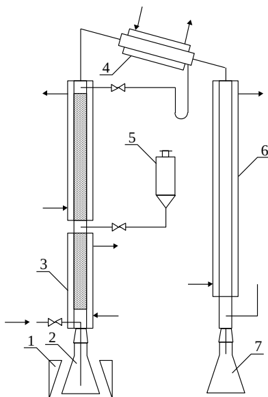
Рис. 3.25. Принципова схема установки для отримання розчинів \text{HNO}_3\text{--N}_2\text{O}_5 : 1 – нагрівач; 2, 7 – приймачі; 3 – ректифікаційна колона; 4 – дефлегматор; 5 – напірна ємність; 6 – холодильник-конденсатор
