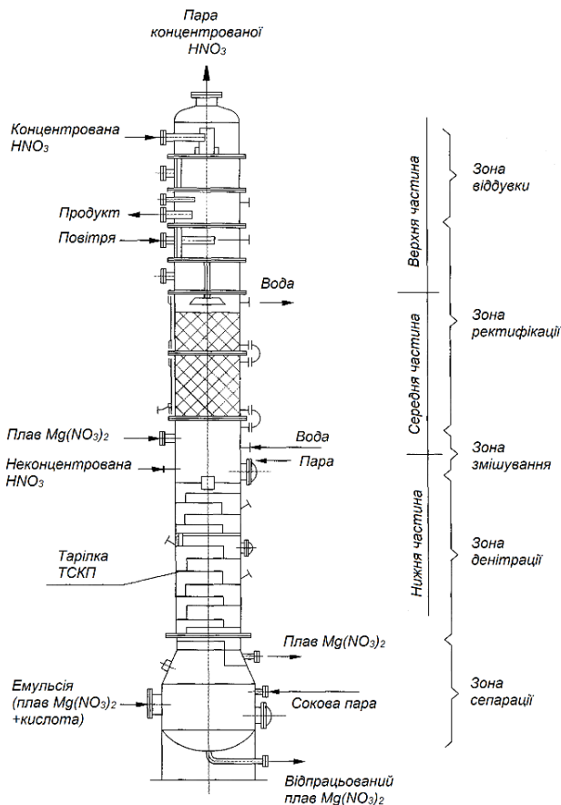
Рис. 5.25. Колона концентрування збільшеної одиничної потужності
