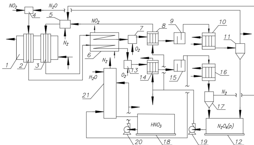
Рис. 5.41. Технологічна схема одержання N_2O та нітратної кислоти з молекулярного N_2 :
