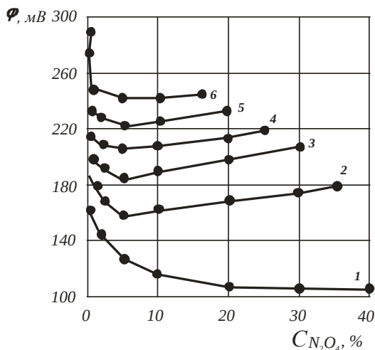
Рис. 3.26. Залежність окиснювально-відновного потенціалу ( \varphi ) розчинів \text{HNO}_3\text{--N}_2\text{O}_5\text{--N}_2\text{O}_4 при 20^\circ\text{C} від концентрації \text{N}_2\text{O}_4 при масовому вмісті \text{N}_2\text{O}_5 , %: 1 – 0,6; 2 – 6; 3 – 12; 4 – 18; 5 – 24; 6 – 30
