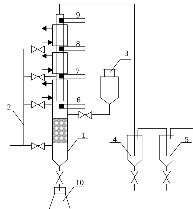
Рис. 3.23. Принципова схема установки для газорідинного окиснення N_2O_4 озono-кисневою сумішшю:
