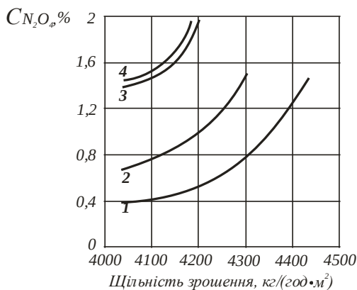
Рис. 3.60. Залежність вмісту N_2O_4 в дистилаті від щільності зрошення при C_{HNO_3} = 98\% мас.; лінійній швидкості пари 0,53 м/с і числах одиниць переносу: 1 – 6; 2 – 7; 3 – 8; 4 – 9
