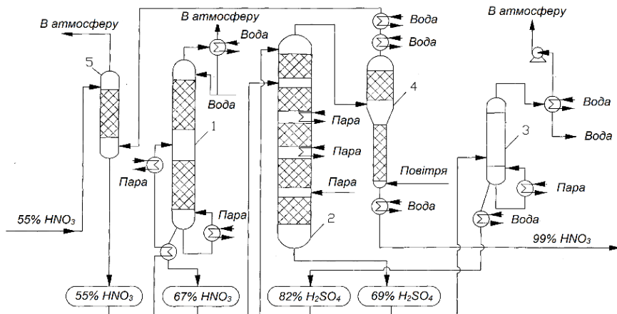
Рис. 5.17. Принципова технологічна схема установки для концентрування нітратної кислоти за способом "ШОТТ":
