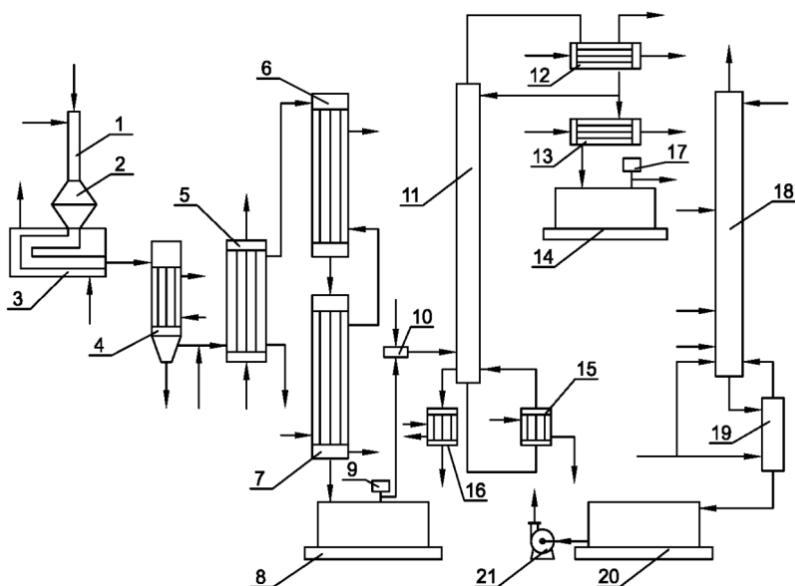
Рис. 5.8. Принципова технологічна схема отримання рідких сумішей \text{N}_2\text{O}_3\text{--N}_2\text{O}_4 методом конденсації оксидів нітрогену з нітрозних газів в складі виробництва неконцентрованої \text{HNO}_3 під тиском 0,8 МПа:
