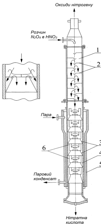
Рис. 5.33. Відбілювальна колона алюмінієва з ситчастими тарілками: 1 – теплообмінна частина (дефлегматор); 2 – каскадні напівтарілки; 3 – ковпачкові тарілки, 4 – нагрівальна частина з кишенями; 5 – стальна сорочка; 6 – ущільнення
