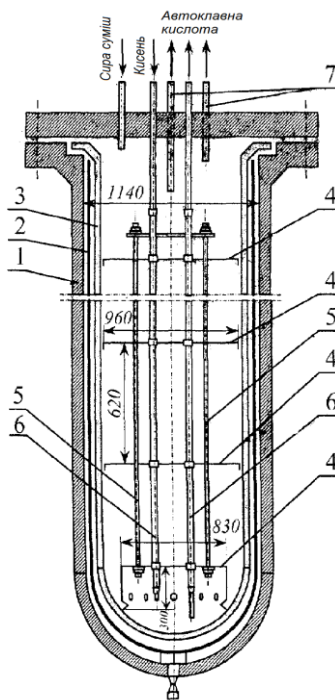
Рис. 5.37. Автоклав з насадкою для одержання концентрованої нітратної кислоти:
