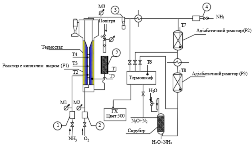
Рис. 5.1. Принципова схема пілотної установки синтезу оксиду динітрогену:
