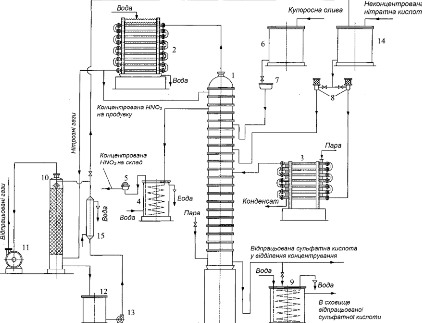
Рис. 5.16. Принципова схема установки для концентрування неконцентрованої нітратної кислоти з допомогою сульфатної кислоти (купоросної оливи): 1 – концентраційна колона; 2 – конденсатор; 3 – випарник розведеної нітратної кислоти; 4 – холодильник концентрованої нітратної кислоти; 5, 8 – контрольний ліхтар; 6 – напірний бак купоросної оливи; 7 – мірник купоросної оливи; 9 – холодильник відпрацьованої сульфатної кислоти; 10 – абсорбційна колона; 11 – газодувка (ексгаустер); 12 – збірник розведеної нітратної кислоти; 13 – відцентровий насос; 14 – напірний бак розведеної нітратної кислоти; 15 – холодильник
