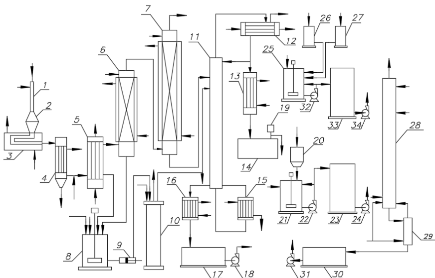
Рис. 5.12. Принципова технологічна схема інгібованих сумішей концентрованої нітратної кислоти та оксидів нітрогену:
