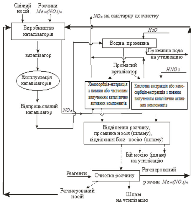
Рис. 6.9. Блок-схема регенерації каталізаторів
