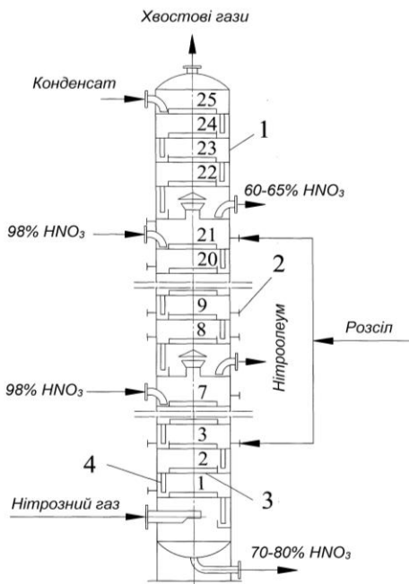
Рис. 5.31. Нітроолеумна колона:
