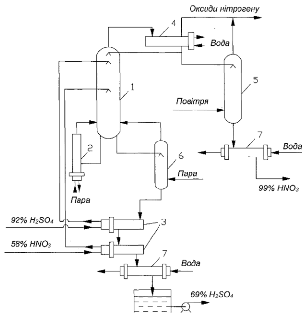
Рис. 5.18. Принципова технологічна схема установки для концентрування нітратної кислоти за способом "Кеметікс":
