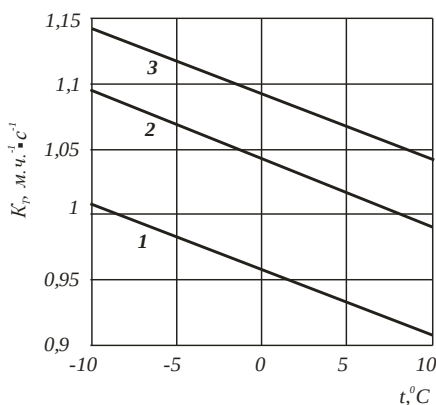
Рис. 3.41. Залежність коефіцієнту швидкості абсорбції від температури при лінійних швидкостях газу, м/с: 1 – 0,2; 2 – 0,4; 3 – 0,6
