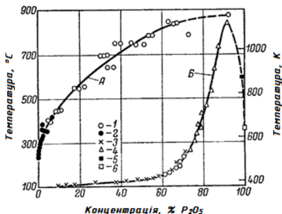
Рис. 1.36. Діаграма температур кипіння і складу пари системи \text{H}_3\text{PO}_4\text{--H}_2\text{O} :
