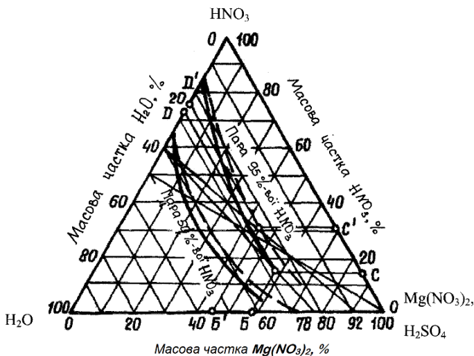
Рис. 5.21. Рівноважна концентрація пари нітратної кислоти над потрійною сумішшю \text{HNO}_3\text{--H}_2\text{O--Mg(NO}_3)_2
