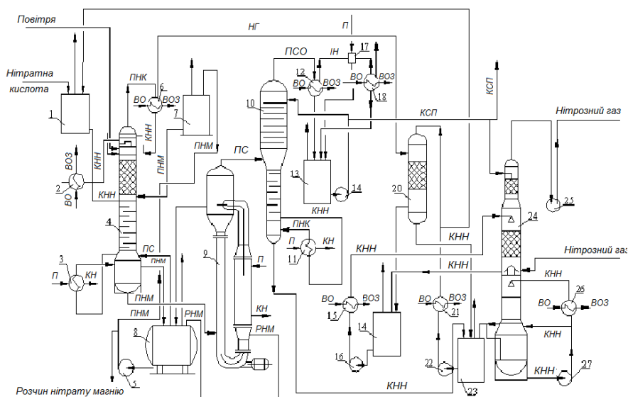
Рис. 5.24. Принципова схема виробництва КНК
