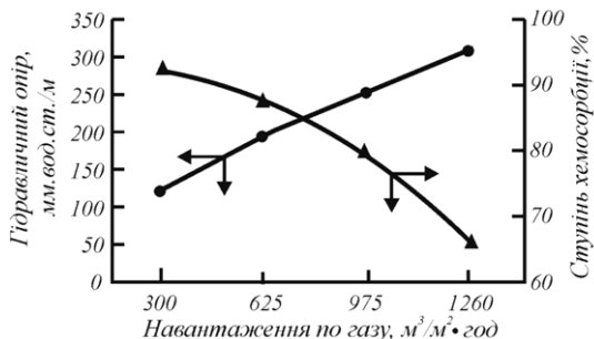
Рис. 6.8. Залежність гідралічного опору та ступеня хемосорбції \text{NO}_x від навантаження по газу при V_p = 9 \text{ м}^3/\text{м}^2 \cdot \text{год}
