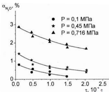
Рис. 4.6. Залежність ступеня окиснення NH_3 в N_2O від часу контактування ( T = 1123 \text{ K} )
