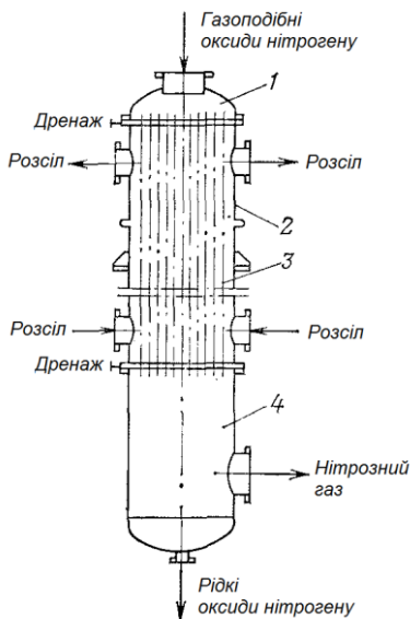
Рис. 5.36. Конденсатор оксидів нітрогену: 1 — кришка; 2 — корпус; 3 — трубки; 4 — сепаратор
