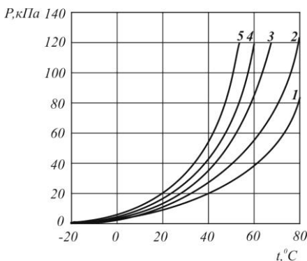
Рис. 3.50. Залежність тиску насиченої пари системи \text{HNO}_3\text{--N}_2\text{O}_5 від температури при концентраціях \text{N}_2\text{O}_5 , %: 1 – 0; 2 – 5; 3 – 10; 4 – 15; 5 – 20
