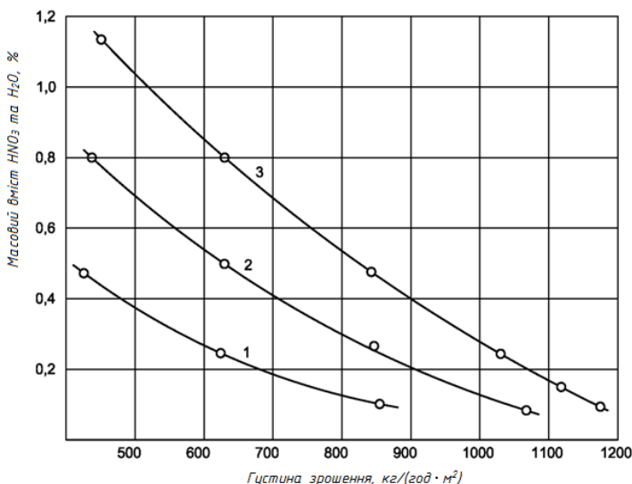
Рис. 3.18. Залежність масового вмісту \text{HNO}_3 та \text{H}_2\text{O} в дистилаті від густини зрошення при початковій концентрації \text{HNO}_3 40% мас., вихідному масовому співвідношенні \text{N}_2\text{O}_4:\text{H}_2\text{O} = 2:1 , лінійній швидкості газу W = 0,125 м/с і різному числі теоретичних тарілок: 1 – 12; 2 – 8; 3 – 4
