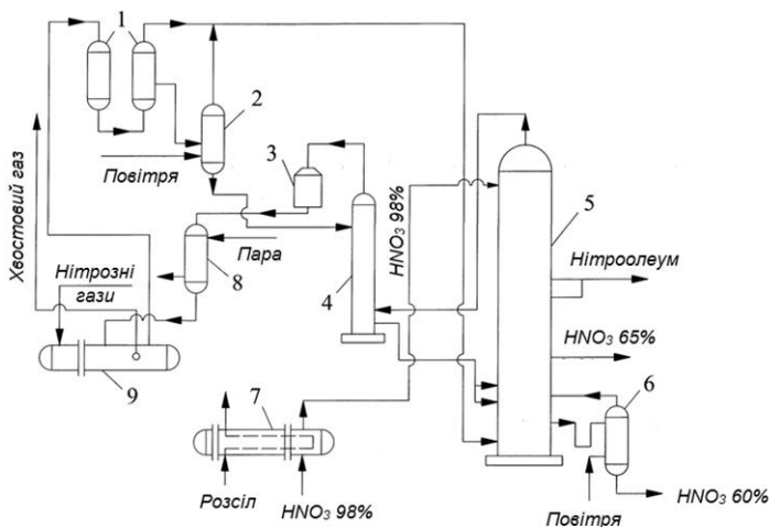
Рис. 5.38. Схема отримання нітролеуму під тиском 0,716 МПа:
