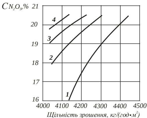
Рис. 3.59. Залежність концентрації N_2O_5 в дистилаті від щільності зрошення при C_{HNO_3} = 98\% мас.; лінійній швидкості пари 0,53 м/с і числах одиниць переносу: 1 – 6; 2 – 7; 3 – 8; 4 – 9
