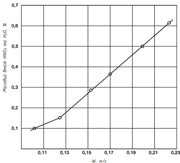
Рис. 3.17. Залежність масового вмісту \text{HNO}_3 та \text{H}_2\text{O} при масовому співвідношенні \text{N}_2\text{O}_4:\text{H}_2\text{O} = 4:1 , густині зрошення 994 \text{ кг}/(\text{год} \cdot \text{м}^2) і числі теоретичних тарілок N = 8
