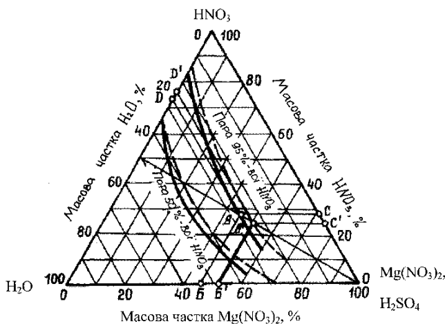
Рис. 5.20. Рівноважна концентрація пари нітратної кислоти над потрійною сумішшю \text{HNO}_3\text{--H}_2\text{O--Mg}(\text{NO}_3)_2 ( \text{H}_2\text{SO}_4 )
