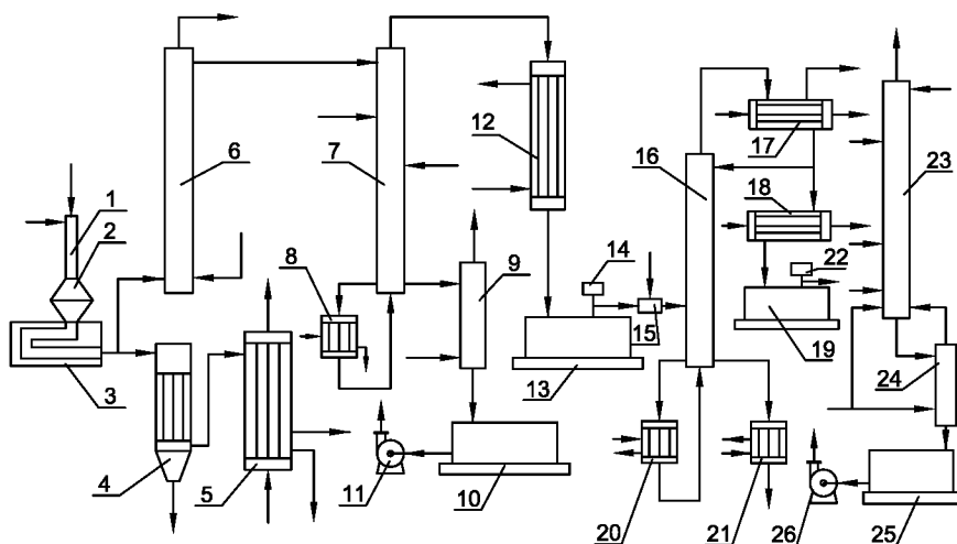
Рис. 5.9. Принципова технологічна схема отримання рідких сумішей N_2O_3-N_2O_4 інверсійних газів в складі виробництва неконцентрованої HNO_3 під тиском 0,8 МПа:
