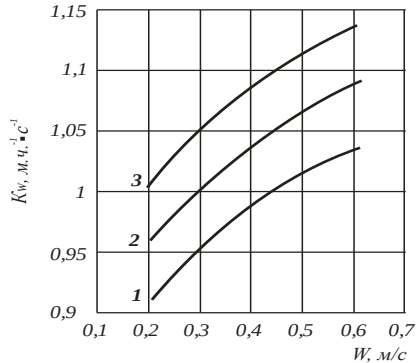
Рис. 3.40. Залежність коефіцієнту швидкості абсорбції від лінійної швидкості газу при температурах, ^\circ\text{C} : 1 – 10; 2 – 0; 3 – ( -10 )
