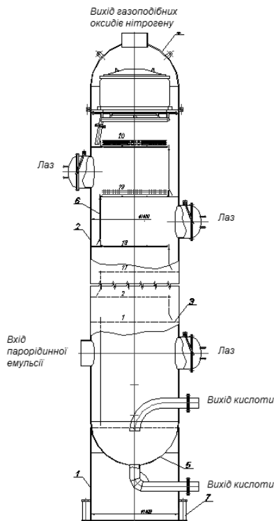
Рис. 5.34. Тарілчаста відбілювальна колона великої потужності:
