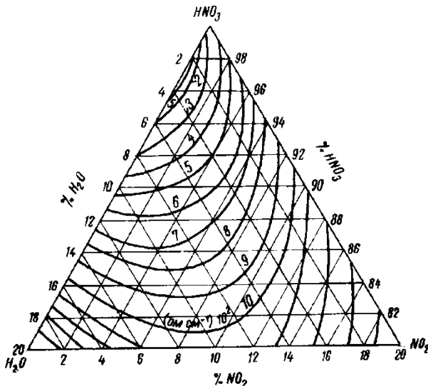
Рис. 1.26. Залежність питомої електропровідності, (\text{Ом} \cdot \text{см})^{-1} , розчинів \text{HNO}_3\text{--N}_2\text{O}_4\text{--H}_2\text{O} від масових концентрацій оксиду нітрогену (IV) та води при 0^\circ\text{C}
