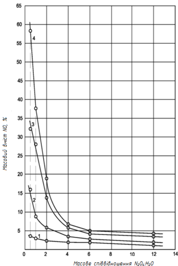
Рис. 3.9. Залежність масового вмісту NO в газовій фазі від масового співвідношення \text{N}_2\text{O}_4:\text{H}_2\text{O} при температурі 303 К та різних масових початкових концентраціях \text{HNO}_3 , %: 1 – 68,4; 2 – 60,3; 3 – 50; 4 – 40
