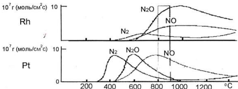
Рис. 4.2. Залежність утворення N 2 O від температури на платині та родії
