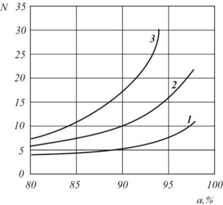
Рис. 3.36. Залежність числа одиниць переносу ( N ) від ступеня поглинання ( \alpha ) N 2 O 5 100%-вою нітратною кислотою при масовому вмісті N 2 O 5 в рідині 30% і температурах, °C: 1 – (–10); 2 – 0; 3 – 10
