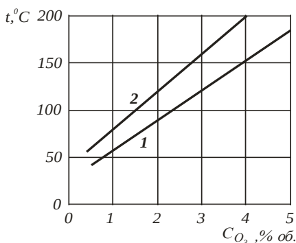
Рис. 3.37. Залежність температури процесу в реакційній камері від початкової концентрації озону в газі: 1 — газорідинне окиснення N_2O_4 ; 2 — окиснення N_2O_4 в газовій фазі
