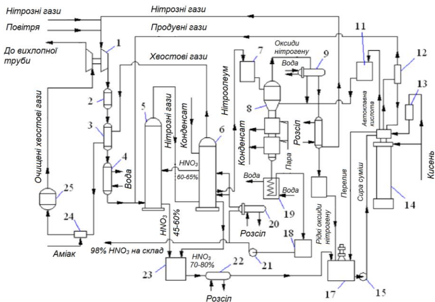
Рис. 5.30. Схема виробництва концентрованої нітратної кислоти методом прямого синтезу при абсорбції оксидів нітрогену під тиском 0,343 МПа:
