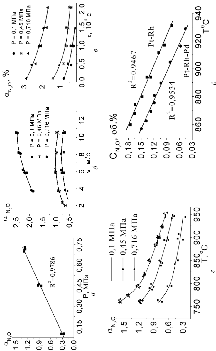
Рис. 3.3. Залежність ступеня перетворення в N_2O в якості побічного продукту при окисненні аміаку на металах платинової групи: a – від тиску; b – від лінійної швидкості; c – від часу контакту; d – від температури на Pt-Rh каталізаторі; d – залежність концентрації N_2O від складу каталізатора
