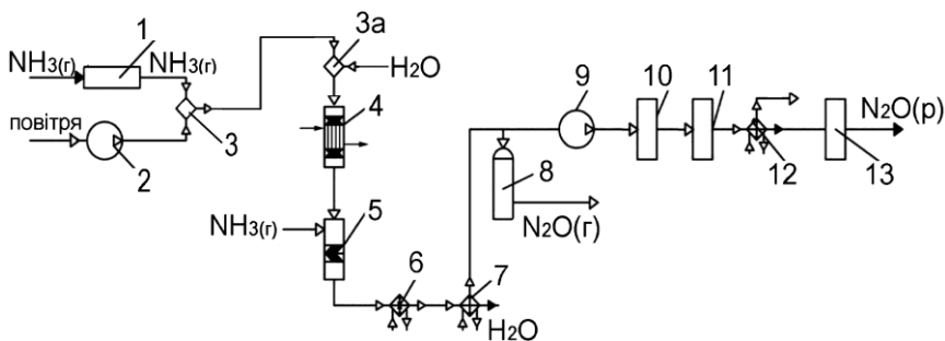
Рис. 3.7. Принципова схема отримання \text{N}_2\text{O} :
