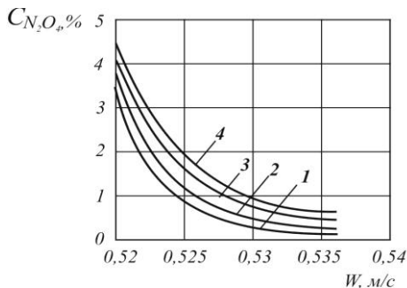
Рис. 3.58. Залежність концентрації N_2O_4 в дистилаті від лінійної швидкості пари при C_{HNO_3} = 98\% мас.; N = 6 і щільності зрошення, кг/(год \cdot м^2) : 1 – 4054; 2 – 4204; 3 – 4299; 4 – 4434
