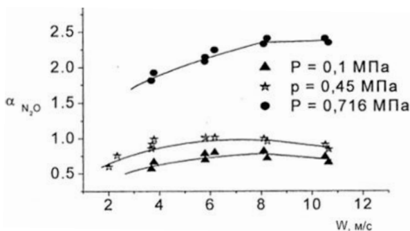
Рис. 4.7. Залежність ступеня окиснення NH_3 в N_2O від лінійної швидкості газу ( T = 850^\circ C )
