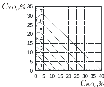
Рис. 3.31. Лінії постійного значення густини (ізодепси) розчинів HNO_3-N_2O_5-N_2O_4 при 0^\circ\text{C} , \text{кг}/\text{м}^3 : 1 – 1560; 2 – 1580; 3 – 1600; 4 – 1620; 5 – 1640; 6 – 1660; 7 – 1670
