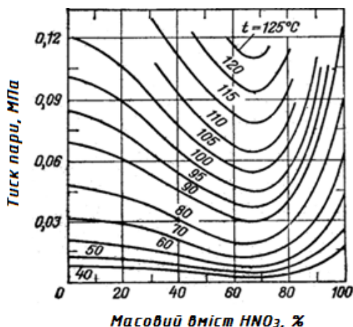
Рис. 1.5. Залежність загального тиску пари над водними розчинами нітратної кислоти при різних температурах
