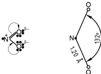
Рис. 1.14. Структура молекули \text{NO}_2
