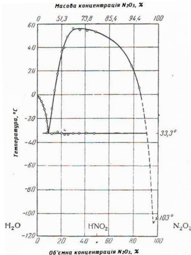
Рис. 1.28. Діаграма розчинності системи \text{N}_2\text{O}_3 – \text{H}_2\text{O}
