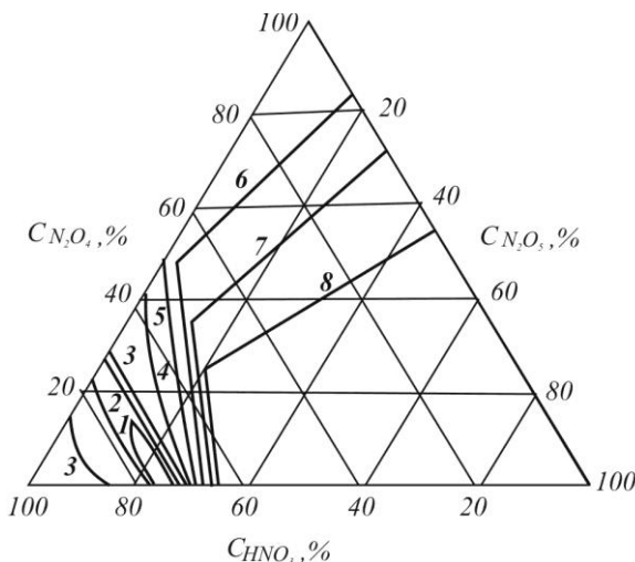
Рис. 3.34. Ізотерми кристалізації розчинів \text{HNO}_3\text{--N}_2\text{O}_5\text{--N}_2\text{O}_4 , °C: 1 – (–70); 2 – (–60); 3 – (–50); 4 – (–40); 5 – (–20); 6 – (–10); 7 – 0; 8 – 10
