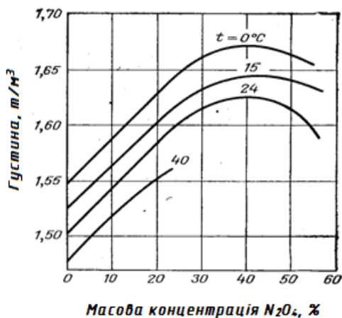
Рис. 1.18. Залежність густини розчинів \text{HNO}_3\text{--N}_2\text{O}_4 від масового вмісту оксиду нітрогену (IV) при різних температурах
