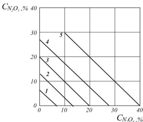
Рис. 3.48. Лінії постійного значення температури кипіння (ізотерми) розчинів \text{HNO}_3\text{--N}_2\text{O}_5\text{--N}_2\text{O}_4 при атмосферному тиску, ^\circ\text{C} : 1 – 70; 2 – 60; 3 – 50; 4 – 40; 5 – 30
