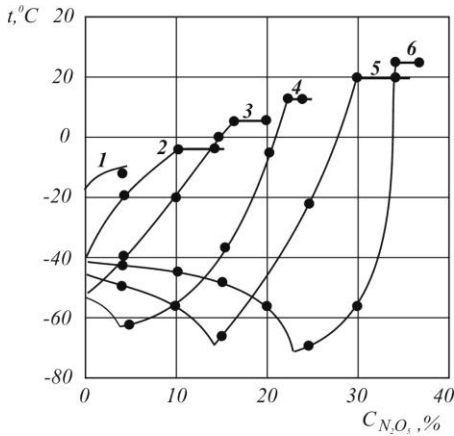
Рис. 3.32. Залежність температури кристалізації розчинів \text{HNO}_3\text{--N}_2\text{O}_5\text{--N}_2\text{O}_4 від масової концентрації \text{N}_2\text{O}_5 при вмісті \text{N}_2\text{O}_4 , % мас.: 1 – 50; 2 – 40; 3 – 30; 4 – 20; 5 – 10; 6 – 0
