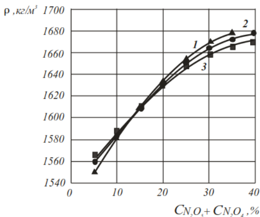
Рис. 3.29. Залежність густини розчинів HNO_3 – N_2O_5 – N_2O_4 від сумарного вмісту оксидів нітрогену при 0^\circ\text{C} і масових співвідношеннях N_2O_5:N_2O_4 : 1 – 30:1; 2 – 10:1; 3 – 1:1
