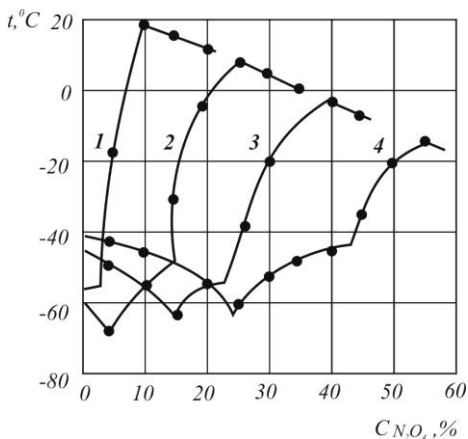
Рис. 3.33. Залежність температури кристалізації розчинів \text{HNO}_3\text{--N}_2\text{O}_5\text{--N}_2\text{O}_4 від масової концентрації \text{N}_2\text{O}_4 при масовому вмісті \text{N}_2\text{O}_5 , %: 1 – 30; 2 – 20; 3 – 10; 4 – 0
