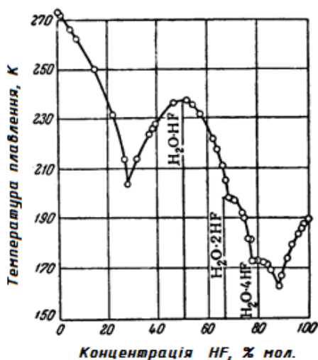
Рис. 1.43. Діаграма плавкості системи HF–H 2 O
