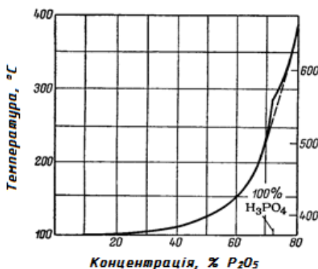
Рис. 1.38. Ізобара системи P_2O_5-H_2O для 101 кПа
