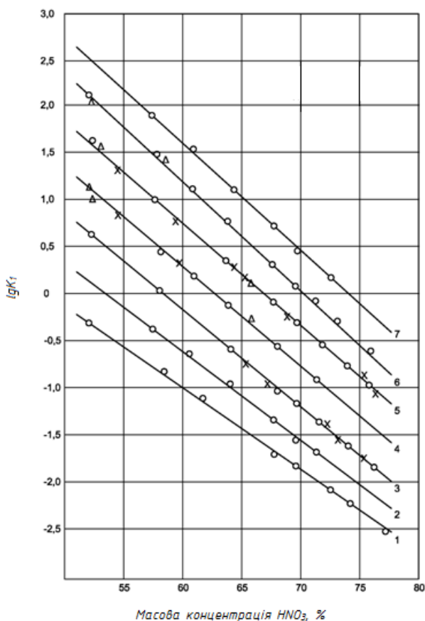
Рис. 3.8. Залежність \lg K_1 від рівноважної концентрації \text{HNO}_3 при різних температурах, К:
