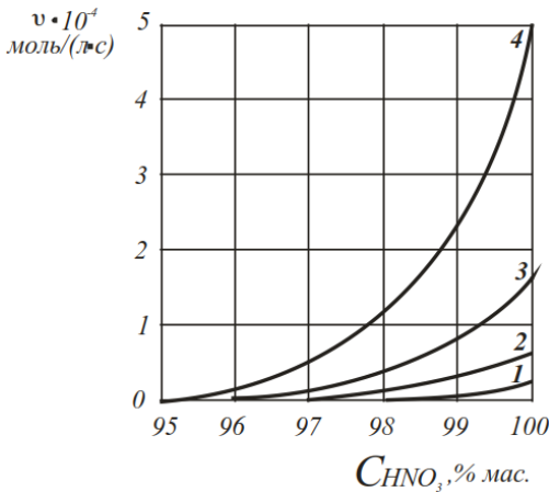
Рис. 3.43. Залежність швидкості розпаду нітратної кислоти від її масової концентрації при t, ^\circ C : 1 – 50; 2 – 60; 3 – 70; 4 – 80
