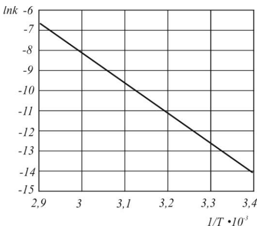
Рис. 3.46. Залежність константи швидкості розкладу розчинів \text{HNO}_3\text{--N}_2\text{O}_5 від температури
