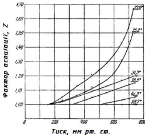
Рис. 1.42. Залежність факторів асоціації HF від тиску при різних температурах
