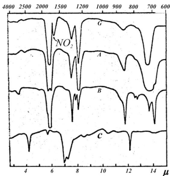
Рис. 1.31. Інфрачервоний спектр пентаоксиду динітрогену
