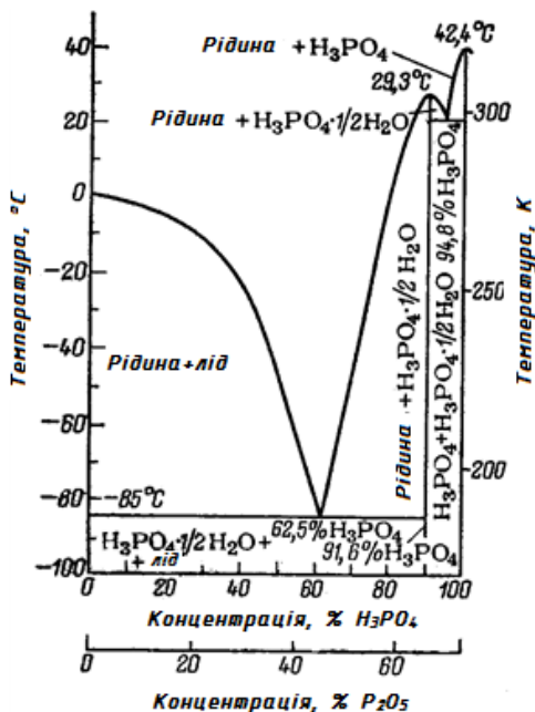
Рис. 1.33. Діаграма стану системи \text{H}_3\text{PO}_4\text{--H}_2\text{O}
