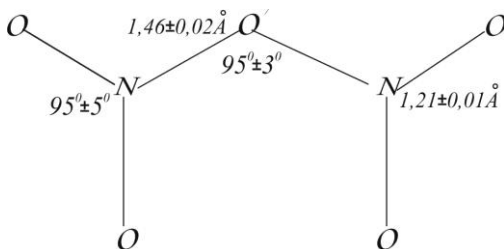
Рис. 1.32. Структура пентаоксиду динітрогену в газовій фазі
