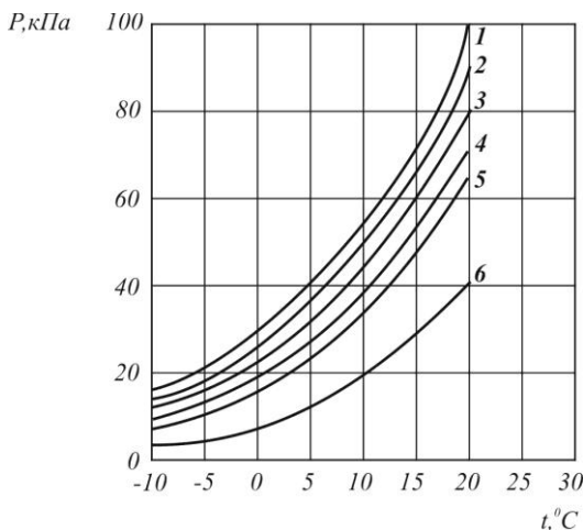
Рис. 3.49. Залежність тиску насиченої пари системи \text{N}_2\text{O}_5\text{--N}_2\text{O}_4 від температури при концентраціях \text{N}_2\text{O}_5 , %: 1 – 0; 2 – 10; 3 – 20; 4 – 30; 5 – 40; 6 – 100
