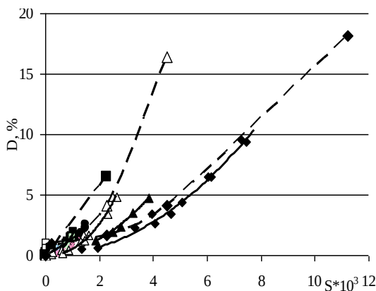
Рис. 6.6. Залежність збільшення рівноважного ступеня перетворення NO_2 за рахунок витрачання нітратної кислоти на екстракцію металів з каталізаторів від S .
