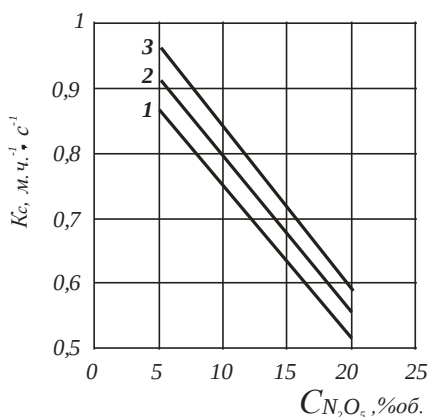
Рис. 3.42. Залежність коефіцієнту швидкості абсорбції від концентрації N_2O_5 в нітратній кислоті при лінійній швидкості газу 0,4 м/с і температурах °C: 1 – 10; 2 – 0; 3 – (–10)
