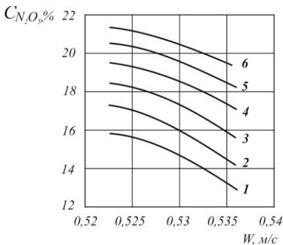
Рис. 3.57. Залежність концентрації N_2O_5 в дистилаті від лінійної швидкості пари при C_{HNO_3} = 98\% мас.; N = 6 і щільності зрошення, кг/(год \cdot м^2) : 1 – 4054; 2 – 4138; 3 – 4204; 4 – 4256; 5 – 4299; 6 – 4434
