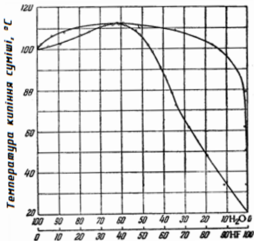
Рис. 1.44. Залежність температури кипіння системи HF–H 2 O від її складу
