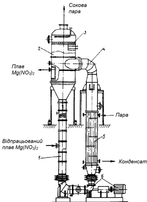
Рис. 5.27. Апарат випарний:
