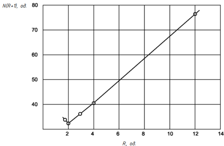
Рис. 3.16. До визначення оптимального значення флегмового числа ( R ) при найменшому об'ємі апарату
