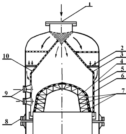
Рис. 3.6. Конструкція реактора з параболоїдними сітками:
