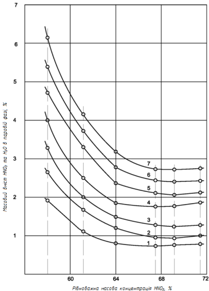
Рис. 3.13. Залежність масового вмісту \text{HNO}_3 та \text{H}_2\text{O} в паровій фазі від рівноважної концентрації \text{HNO}_3 в рідкій фазі при початковій масовій концентрації нітратної кислоти 50% і температурах, К:
