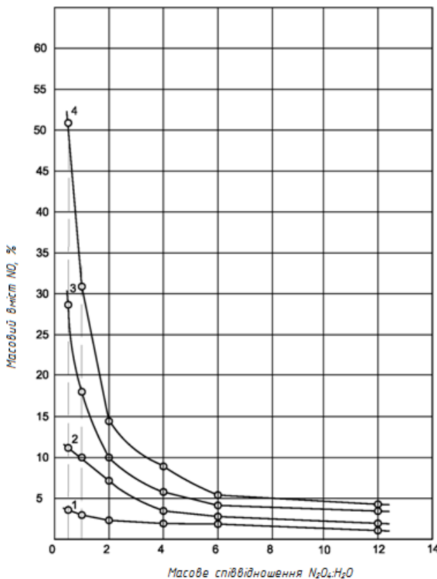
Рис. 3.12. Залежність масового вмісту NO від N_2O_4:H_2O при температурі 303 К та різних масових початкових концентраціях HNO_3 , %: 1 – 68,4; 2 – 60,3; 3 – 50; 4 – 40
