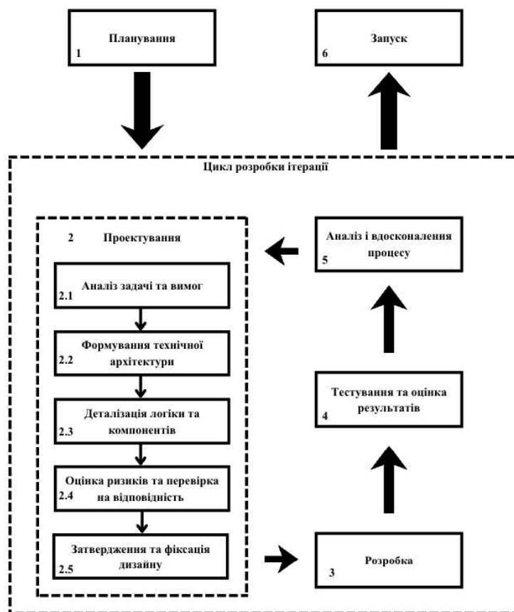
Рисунок – Метод раннього виявлення відхилень в Agile
