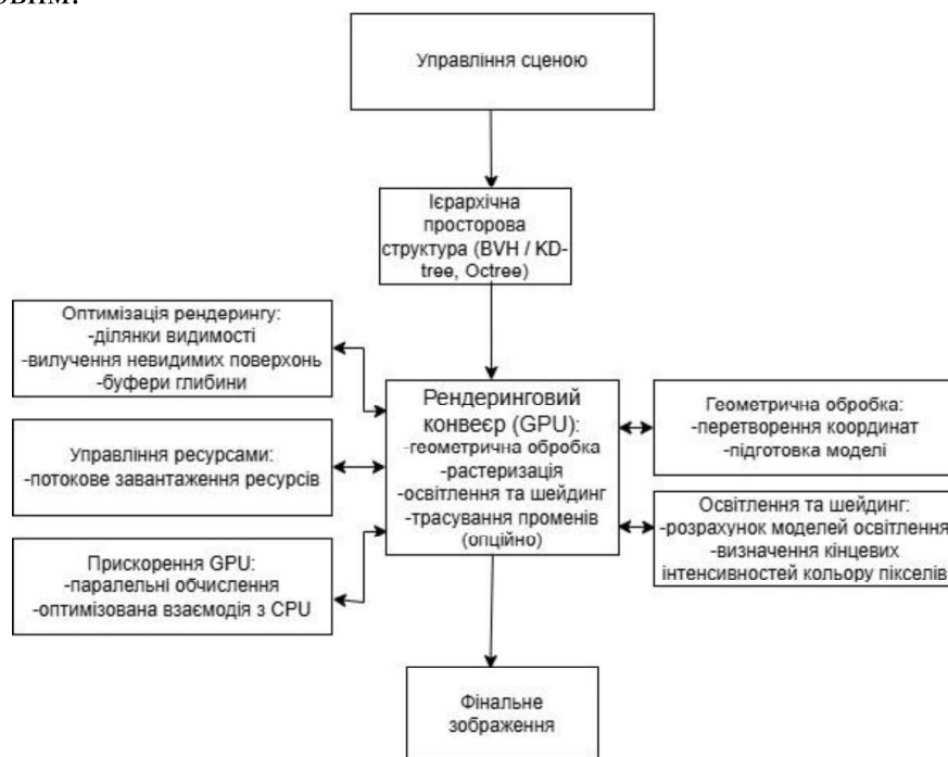
Рисунок – Типова архітектура системи для 3D-рендерингу великих сцен
