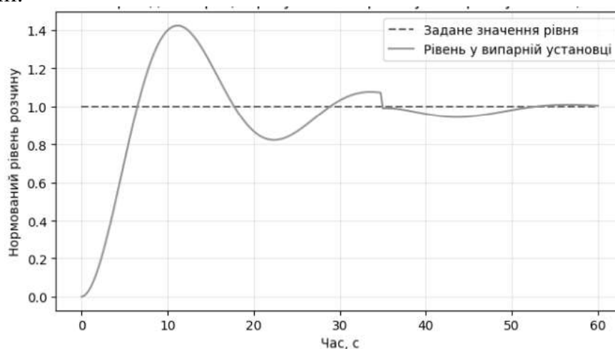
Рисунок — Перехідний процес регулювання рівня у випарній установці
