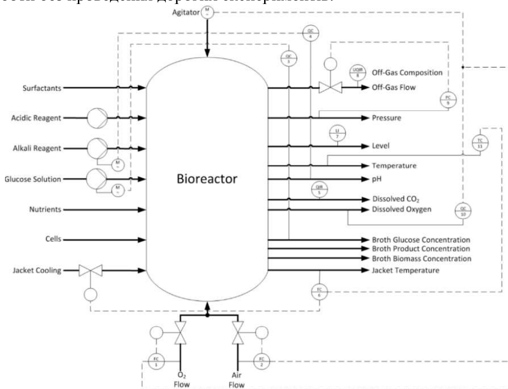
Рисунок – Структурна схема автоматизованої системи управління ферментером
