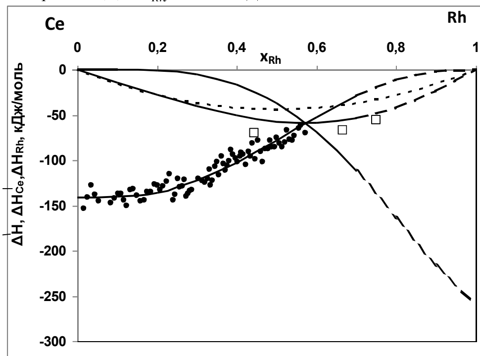
Рис. 1. Парціальні та інтегральні ентальпії змішування розплавів системи Се-Rh при T = 1773\text{ K} .
