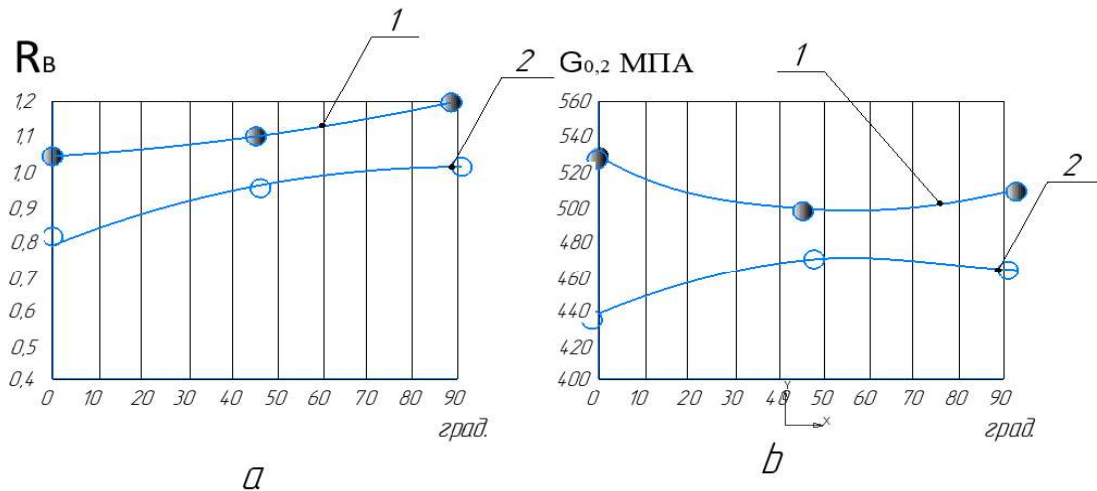
Рисунок 1. Залежності зміни коефіцієнтів анізотропії R_{\beta} (а), меж пластичності \sigma_{0.2\beta} (б) від кута вирізки зразків
