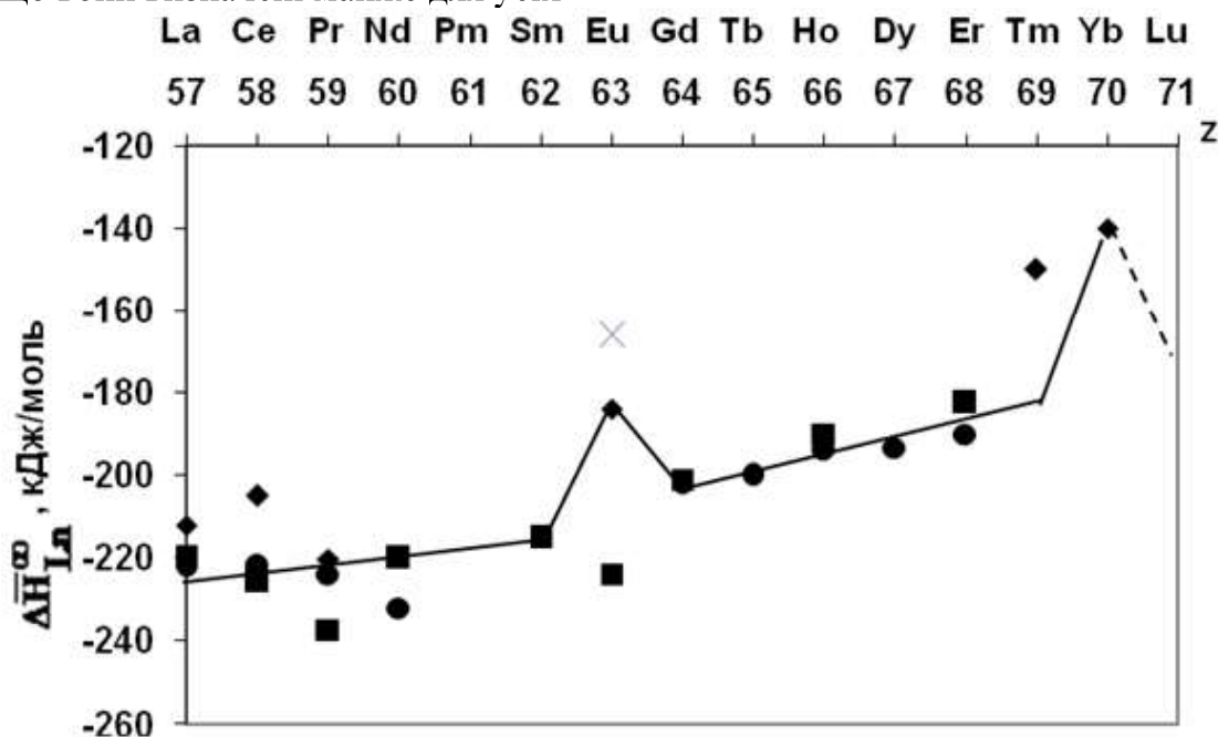
Рисунок 2 – Перші парціальні ентальпії змішування Ln в розплавах систем Bi–Ln за нашими даними при T = 1220 \pm 1\text{K} і вивченими методом ЕРС при 800–1100K (точки – наші і літературні дані)
